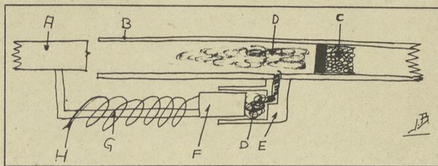
A - culasse mobile B - canon C - bourre et charge de plombs, ou pour une carabine la balle D - gaz de combustion E - conduit et support du cylindre F - piston G - levier d'armement H - ressort de récupération.
