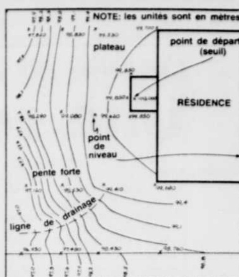
DESSIN NO 2: Plan de la topographie existante
