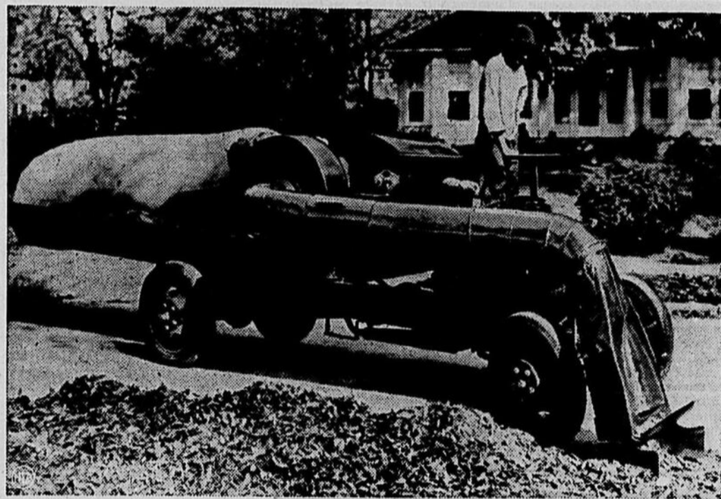
Voici une drôle de machine appelée à acquérir une vogue immense. Il s'agit, en effet, d'une ramasseuse de feuilles mortes que son inventeur, Fred Gedge, du Wyoming, est en train de démontrer. Il l'a entièrement construite avec un vieux camion, un vieux moteur, un vieil éventail, un vieux tuyau, enfin avec beaucoup de vieilles choses. Sa popularité lui viendra sans doute du peu de goût éprouvé par à peu près tout le monde à faire la cueillette des feuilles mortes.
