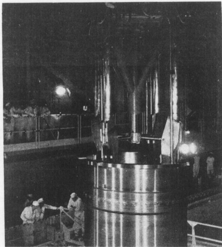
2- Notre photo montre le réacteur atomique installé dans une usine de la Pensylvanie.
