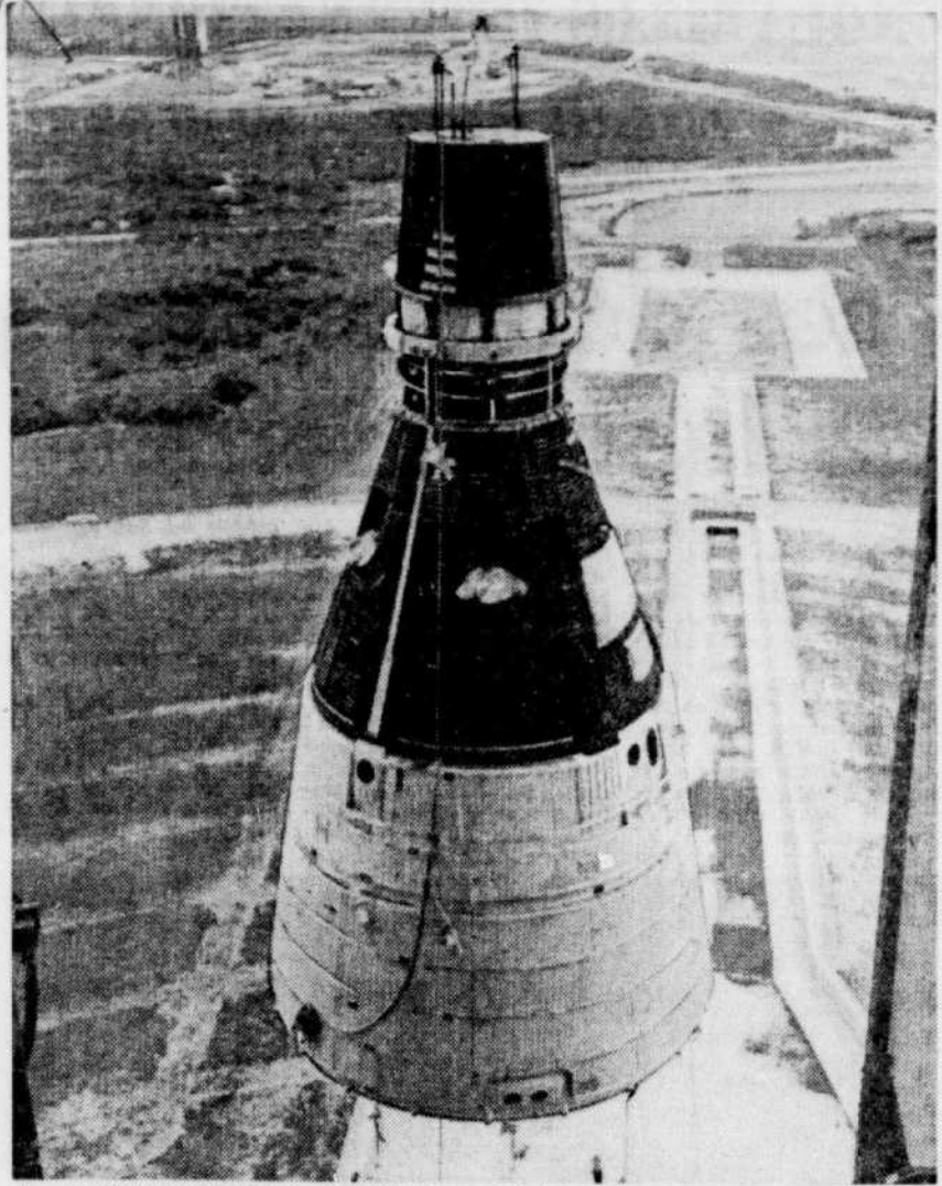
LE VAISSEAU SPATIAL GEMINI 1, qui doit être lancé la semaine prochaine est soulevé pour qu'on l'ajuste à la fusée porteuse Titan II. Après des mois de retard, l'Agence américaine de l'Espace a annoncé qu'elle tenterait la semaine prochaine de placer sur orbite un vaisseau spatial inhabité. Cet essai, qu'un autre suivra, devrait permettre ensuite d'envoyer dans l'espace deux hommes à bord du même vaisseau spatial.
