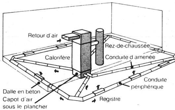
Calorifère à air chaud fonctionnant par gravité
