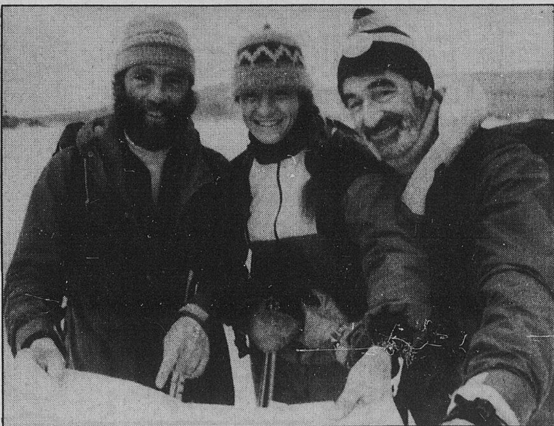
Comme ils le font à tous les jours depuis maintenant plus d'un mois, Vallier Bouchard, Martine de Zwiré et Pierre Gougoux, trois des 32 membres de l'expédition Jacques-Cartier, consultent la carte sur laquelle est tracé leur parcours de 1,600 km de Gaspé à Hull. Les skieurs doivent arriver à Hull dimanche après être partis de Gaspé le Jour de l'An.
