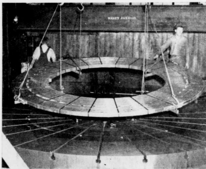
Une des bobines d'aluminium est soulevée de la machine à l'usine de Lachine de la Dominion Engineering.
