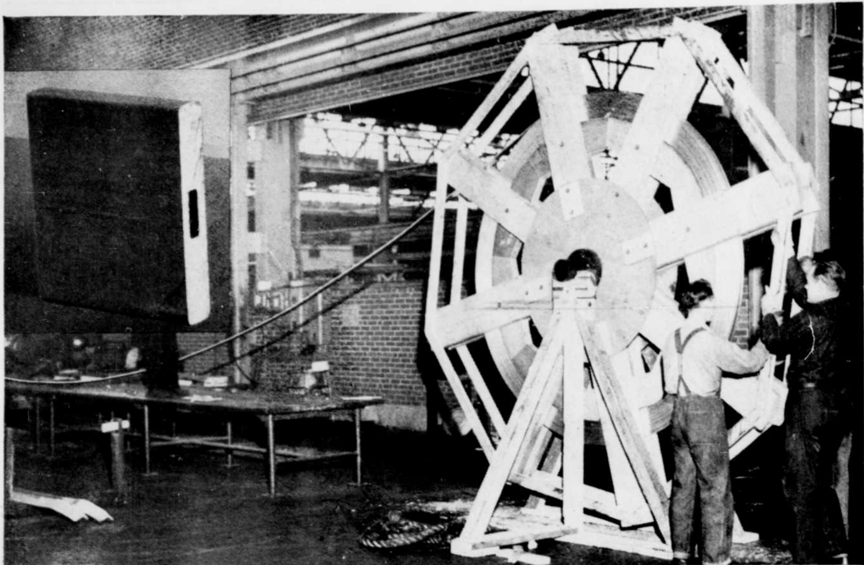
La photo ci-dessus montre l'un des conducteurs extrudés de 1650 pieds de longueur sans qu'il y ait de soudure. On le voit sortir des presses à notre usine de Kingston alors qu'on est en train de l'enrouler sur un tambour pour l'envoyer à la Dominion Engineering Works à Montréal. L'insertion montre une section de cette extrusion continue.
