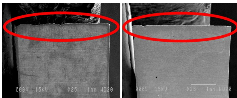
Figure 5 : Arête tranchante d'une dent de scie circulaire normale (gauche) et modifiée (droite) après quatre heures de fonctionnement
