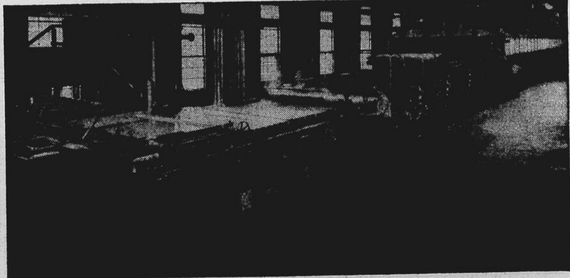
Vue d'ensemble d'une machine à papier. La pâte est introduite à l'extrémité droite et le papier se forme à mesure que la matière se rapproche de l'autre extrémité où il s'enroule sur un cylindre. (gracieuseté de la compagnie de Papier Rolland)
