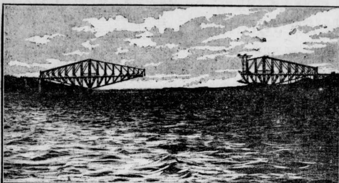
LE PONT DE QUEBEC.—Cette photographie, la plus récente qui soit, représente l'état actuel des travaux au pont de Québec; c'est là une vue prise en regardant vers l'est.
