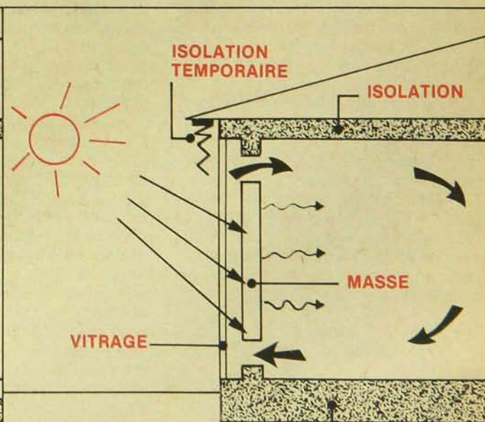
Le mur Trombe ne sera vraiment efficace qu'avec une isolation temporaire de la paroi vitrée pendant les périodes sombres.
