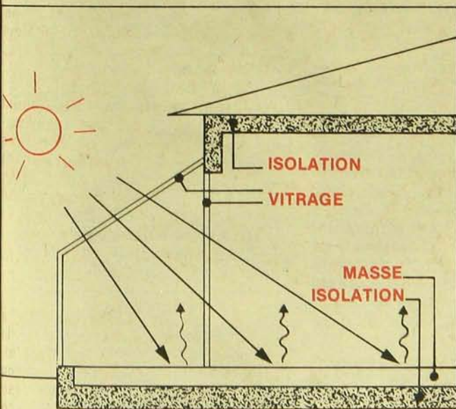
Une serre attenante prolongeant la porte patio offre un gain direct de chaleur et un espace tampon avec l'extérieur.
