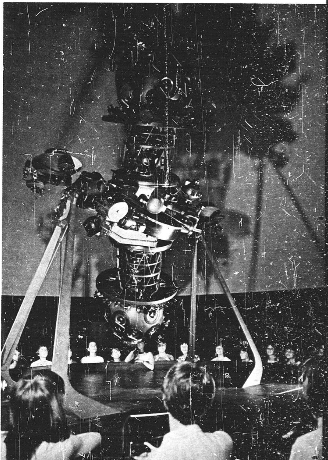
Telle une monstrueuse machine, le projecteur Zeiss domine l'assistance des curieux venus voir les spectacles d'astronomie. ◀
