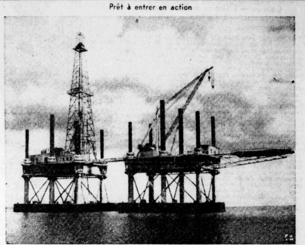
Cet outillage mobile et devant servir à tirer l'huile du fond de la mer, a été construit à Beaumont, Tex. Il sera utilisé dans le golfe du Mexique et peut travailler dans 100 pieds d'eau.
