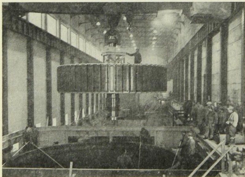
Et, à chaque turbine, on attela une puissante génératrice.
