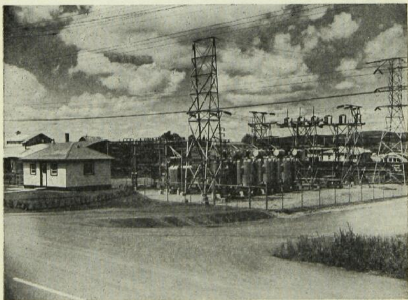
Le poste de transformation de la compagnie Shawinigan à Thetford-Mines. Son rôle consiste simplement à abaisser la tension du courant reçu pour alimenter les consommateurs locaux.
