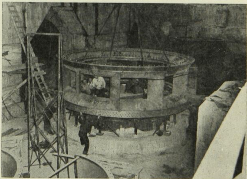
On installa les turbines, dans lesquelles l'eau devait tomber d'une hauteur de 160 pieds.
