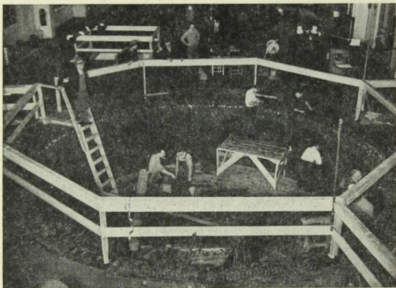
Le rebobinage d'une turbine dans une centrale de la compagnie Shawinigan.
