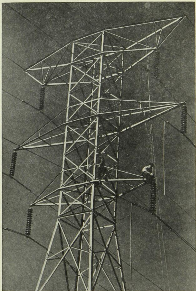
Les gardes-lignes sont habitués à travailler au sommet des pylônes de grande ligne comme en haut des poteaux de petite ligne.
