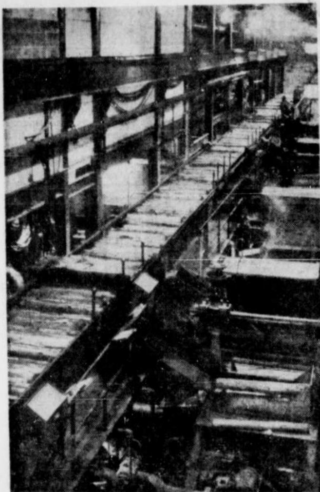
Les pièces de bois s'avancent et tombent contre les meules "Electric Grinder" qui les transforment aussitôt en une pâte humide qui servira à la fabrication du papier à journal.
