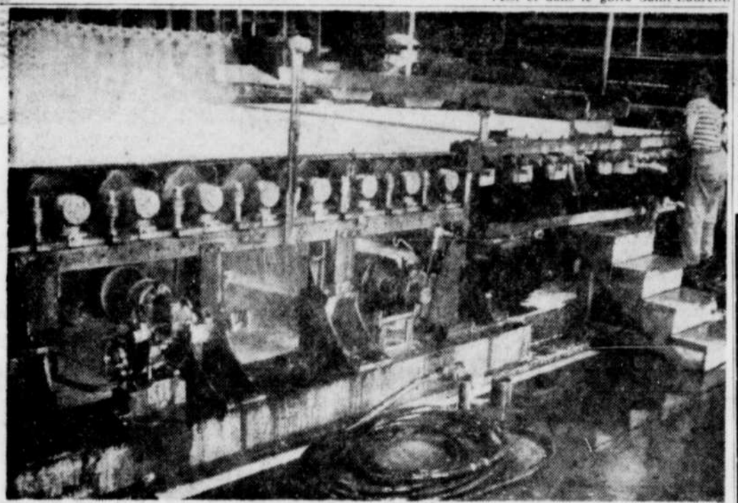
La pâte tombe sur une couverture laineuse qui l'assèche et lui donne le fini que l'on connaît du papier. Les dernières opérations de cuisson termineront le travail de fabrication du papier à journal.
