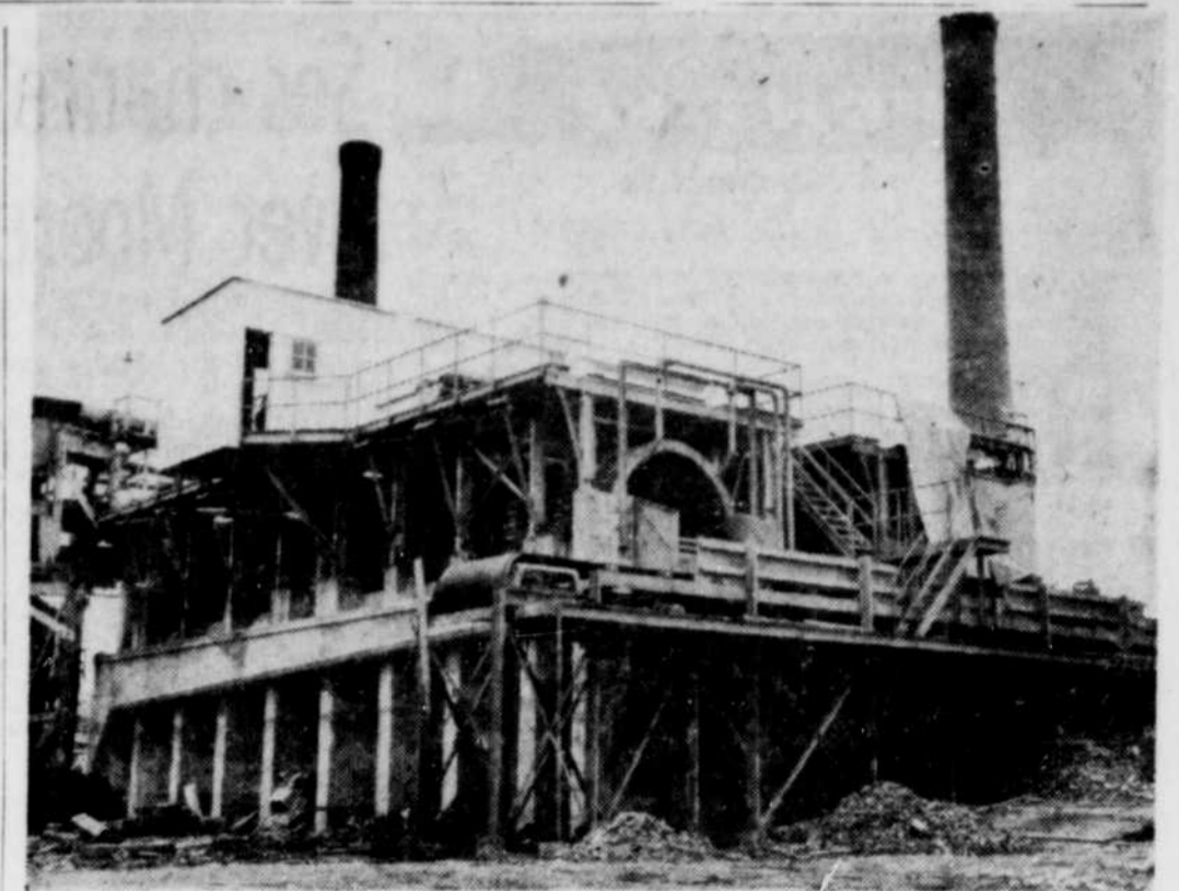
L'écorçage est la première opération que subit la pièce de bois. Voyageant sur convoyeur, elle est portée aux couteaux qui la débarrasse de son écorce.
