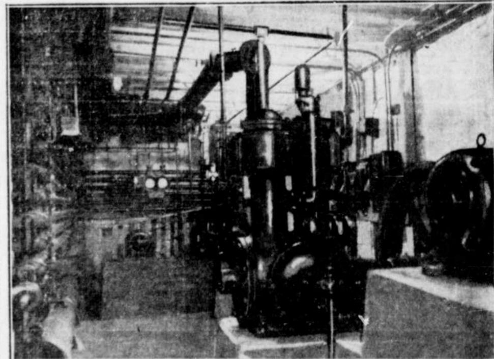
L'entreposage frigorifique des oeufs et des volailles exige un système de réfrigération touz à fait important. L'on voit ici une partie des machines employées à cet effet.
