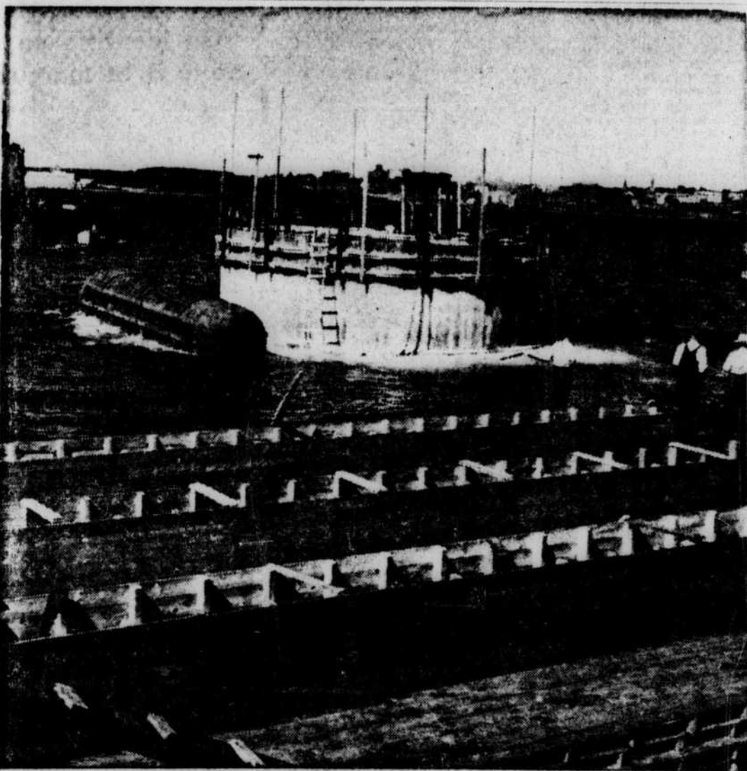
UN CAISSON DE 200 TONNES. — On vient de lancer à l'eau cet énorme caisson de la plate-forme où on l'avait construit. La scène s'est déroulée à Woodside, près de Halifax. Il appartient à une compagnie d'huile. Des ouvriers en feront un pilier qui supportera les poutres en béton armé et les dalles de ciment d'un quai. (Photo CP)
