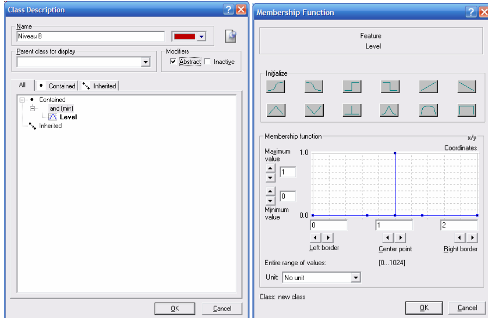
Figure 9. Description de la classe « Niveau B » qui assure la classification des objets du Niveau 1 selon les règles définies pour les classes uniquement de ce niveau. (La description des classes « Niveau H » et « Niveau M » est analogue)
