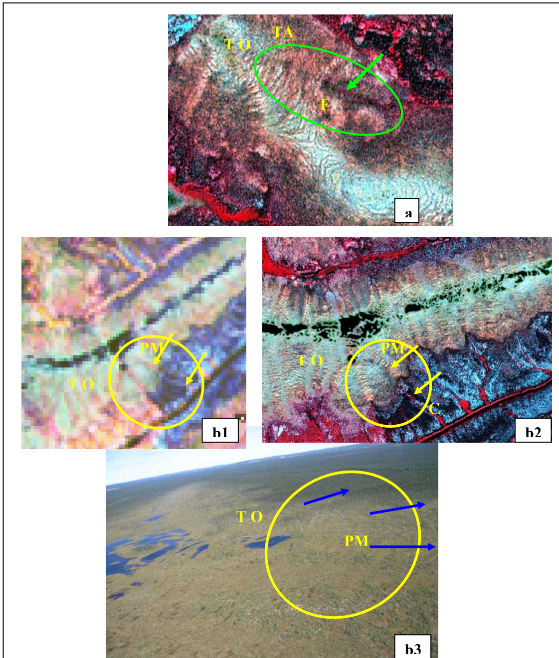
Figure 29. Sites potentiels de connectivité physique. (a) Image QuickBird d'une tourbière ombrotrophe. L'écoulement est plus évident dans la partie plus arborée (FT), ce qui suggère un écoulement sous la surface dans la tourbière ombrotrophe (TO); (b1) Image Landsat-7 ETM+ d'une tourbière ombrotrophe. Les parties en rose dans les limites de la tourbière ombrotrophe (TO) sont des parties plus humides et enrichies en minéraux (PM), ce qui signifie que ce sont les endroits où l'écoulement converge; (b2) Image multispectrale QuickBird du même site que (b1) – évidemment cette image est plus sensible pour les zones d'évacuation des eau (C) hors les limites de la tourbière et moins sensible que l'image Landsat-7 ETM+ pour les zones PM car le capteur QuickBird ne dispose pas de bande dans le MIR ; (b3) la vue aérienne du même site que (b1) et (b2).
