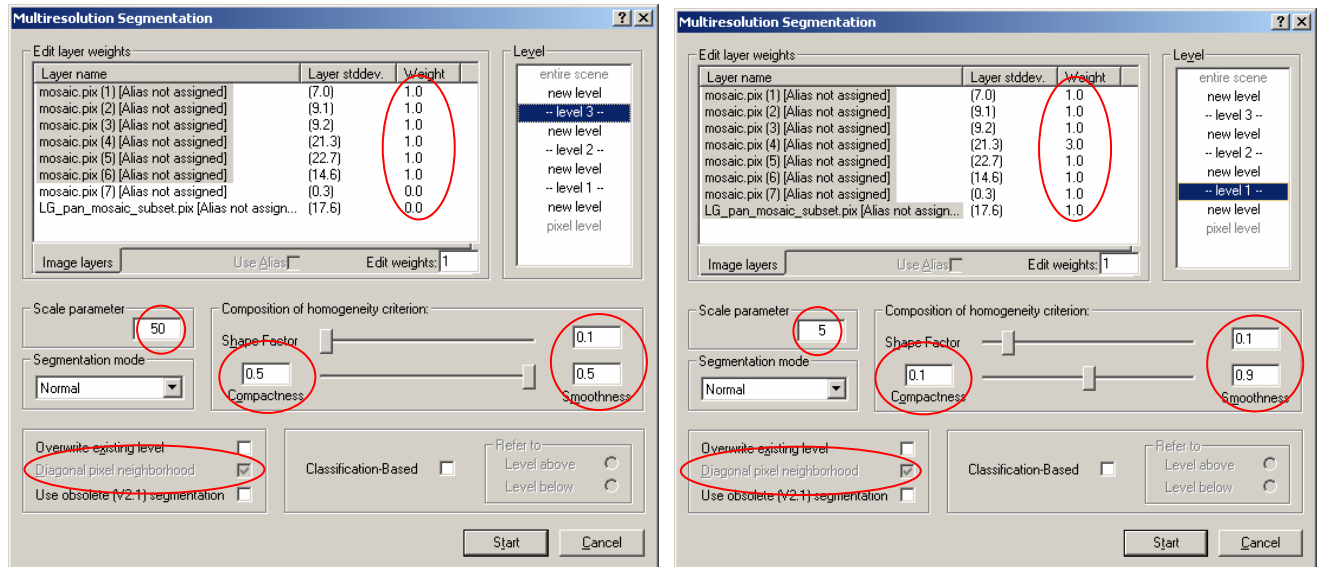
Figure 8. Paramètres de segmentation de Niveau 3 (level 3) et du Niveau 1 (level 1).
