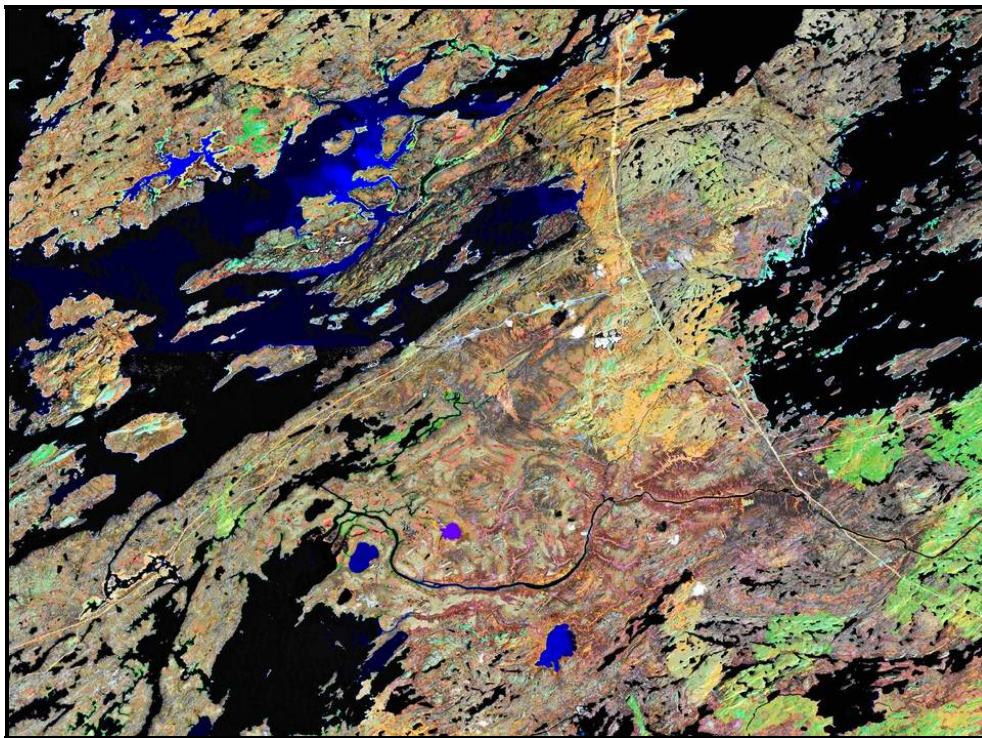
Figure 2. Sous-image du secteur LG-3 (Source : Landsat-7 ETM+; composée couleur RVB – PIR/MIR/V).
