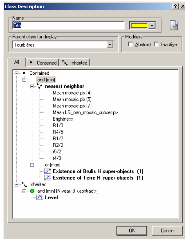
Figure 12. Description de la classe « Fen » du niveau plus fin (Niveau B).
