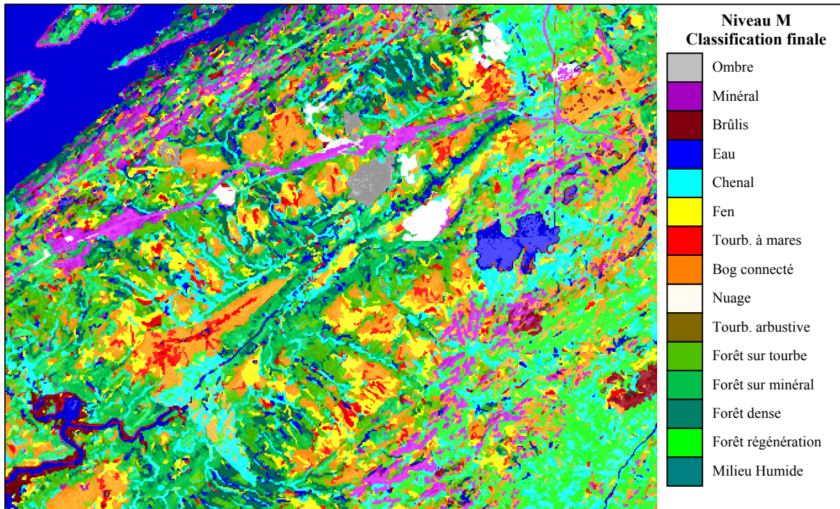
Figure 18. Classification orientée-objet de la zone B (sous-image du secteur LG-3; Niveau M).
