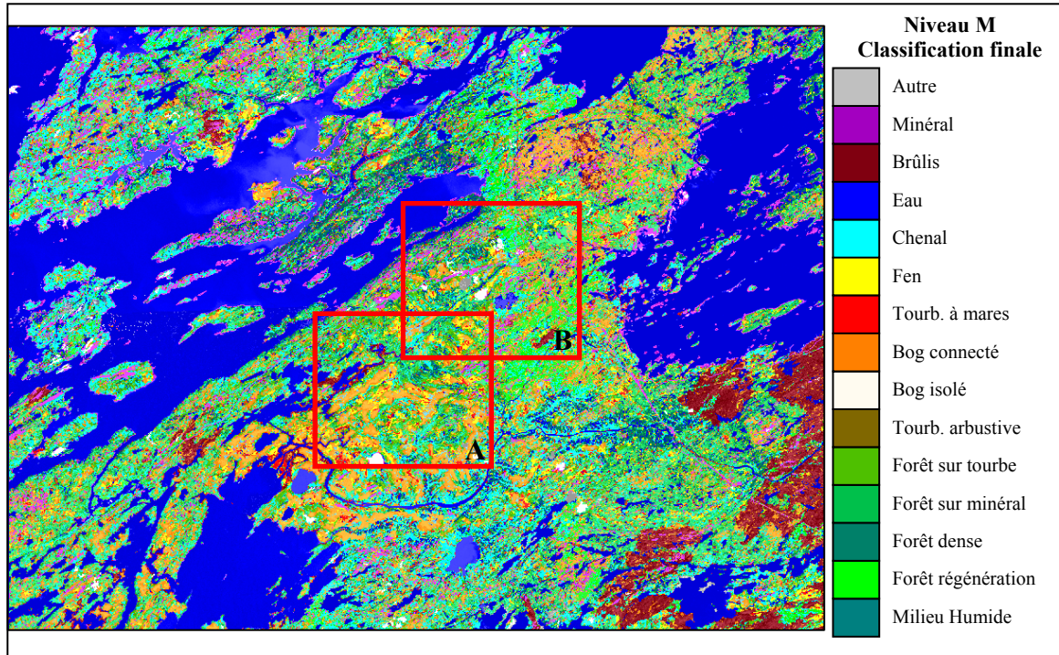
Figure 16. Classification orientée-objet de la sous-image du secteur LG-3 (Niveau M).
