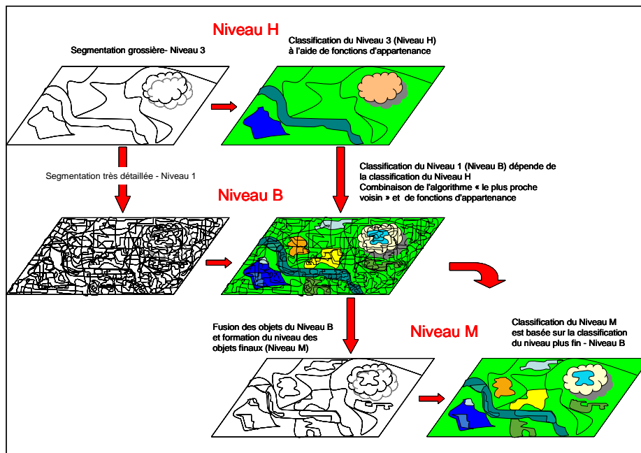
Figure 10. Schéma de la méthode
