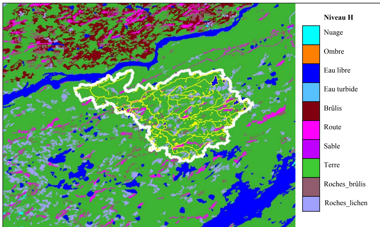
Figure 19. Classification orientée-objet du sous-bassin de la rivière Nécopastic (Niveau H).
