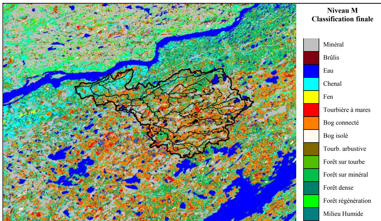
Figure 20. Classification orientée-objet du sous-bassin de la rivière Nécopastic (Niveau M).
