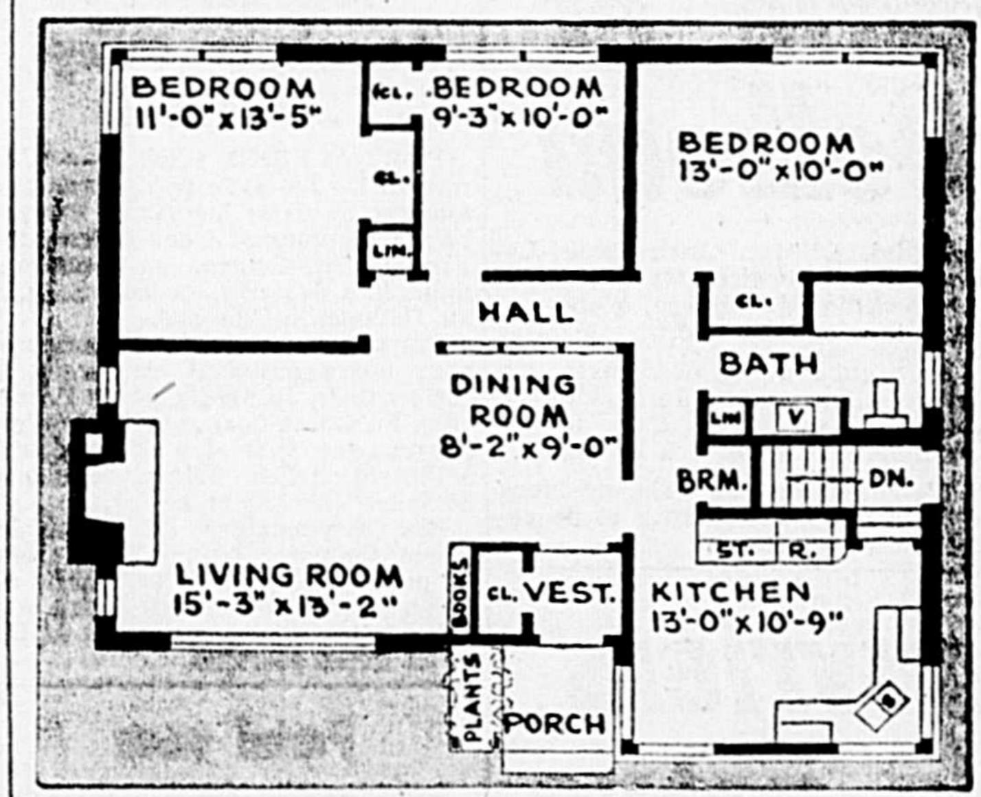
UNE GRANDE PIÈCE pour la salle de séjour et la salle à manger occupe tout l'avant gauche de ce modèle et il y a un petit espace pour la table de goûter dans la cuisine. Les chambres à coucher sont à l'arrière de la maison.
