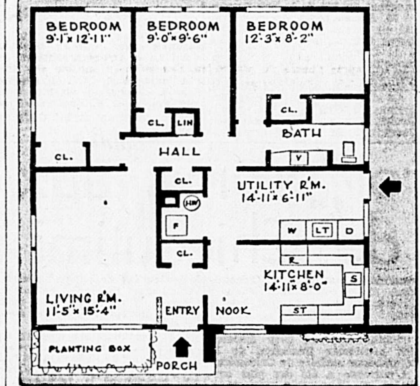
IL N'Y A PAS D'ESPACE PERDU dans ce plain-pied, qui comprend trois chambres à coucher, une salle de bain, une salle de séjour, une salle d'utilité et la cuisine.
