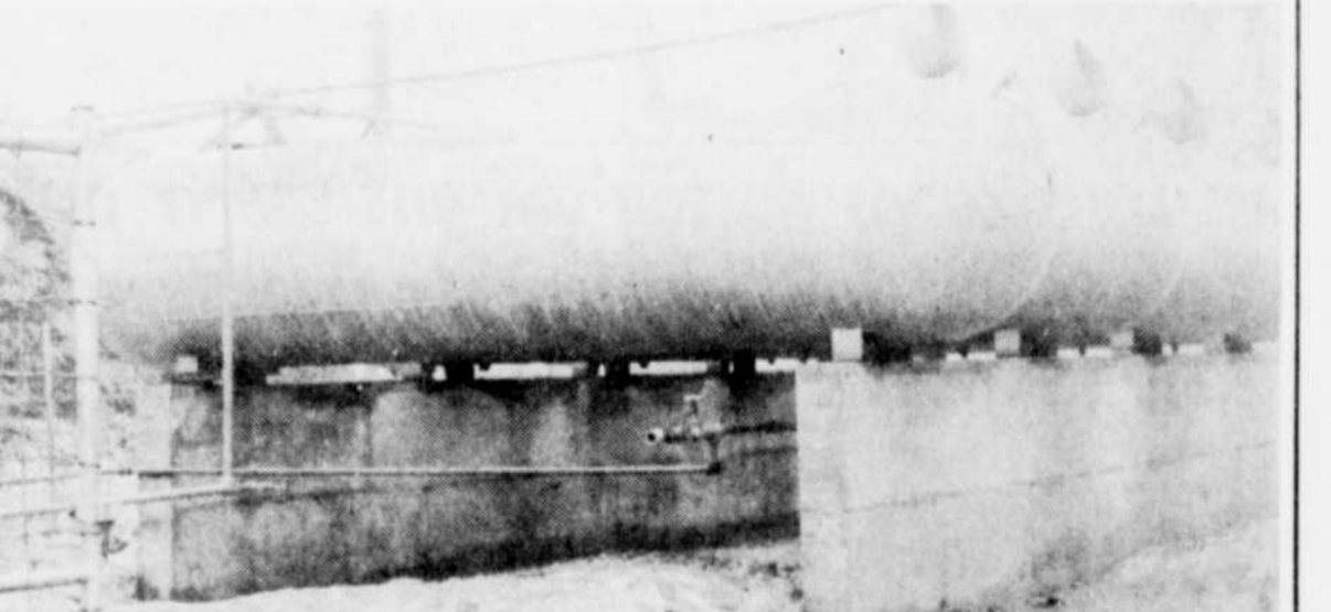
LE COMBUSTIBLE — Le gaz propane qui alimente la fournaise provient de six imposantes bonbonnes d'une capacité de 1,750 gallons chacune. (Photo La Tribune, Thetford Mines)
