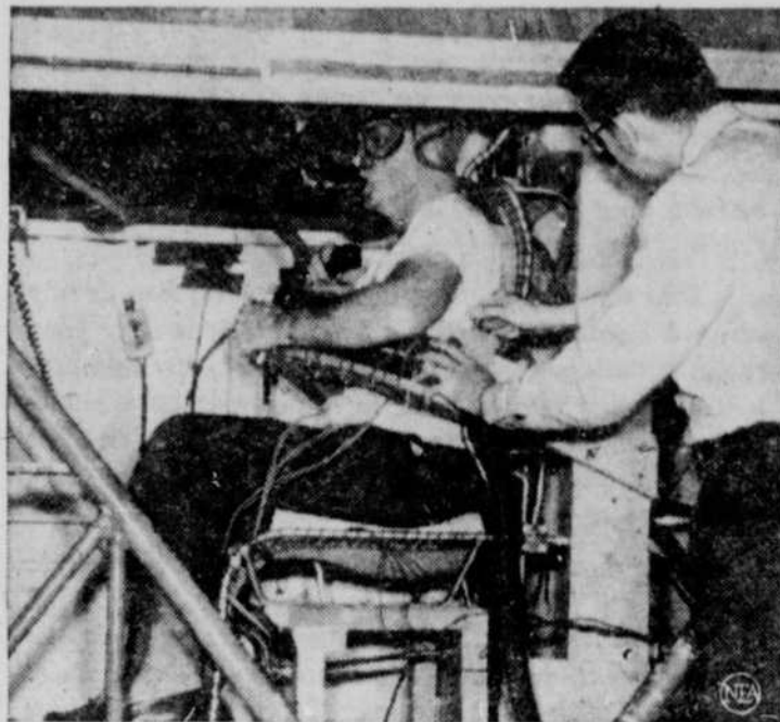
GRAVITE : Le candidat doit supporter aussi les effets de la gravité. Le lieutenant-colonel de marine John H. Glenn, Jr., se prépare à subir les effets de l'accélération et à cette fin, on le fait tourner dans un appareil imitant les mouvements du centrifuge.
