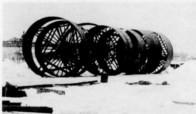
Quelques-unes des pièces de dix pieds de longueur et de vingt-trois pieds de diamètre qui sont déjà prêtes. Fabriquées avec des feuilles de métal de un pouce et demi d'épaisseur, elles pèsent vingt-trois tonnes chacune... (Photo P.E., J. Gédéon)
