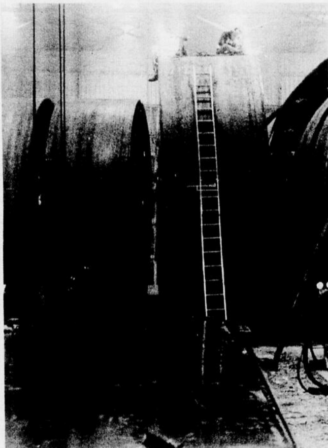
Cette photo nous permet de nous faire une idée du format des pièces; les soudeurs à l'oeuvre sont petits, comparés aux cylindres sur lesquels ils travaillent... (Photo P.E., J. Gédéon)
