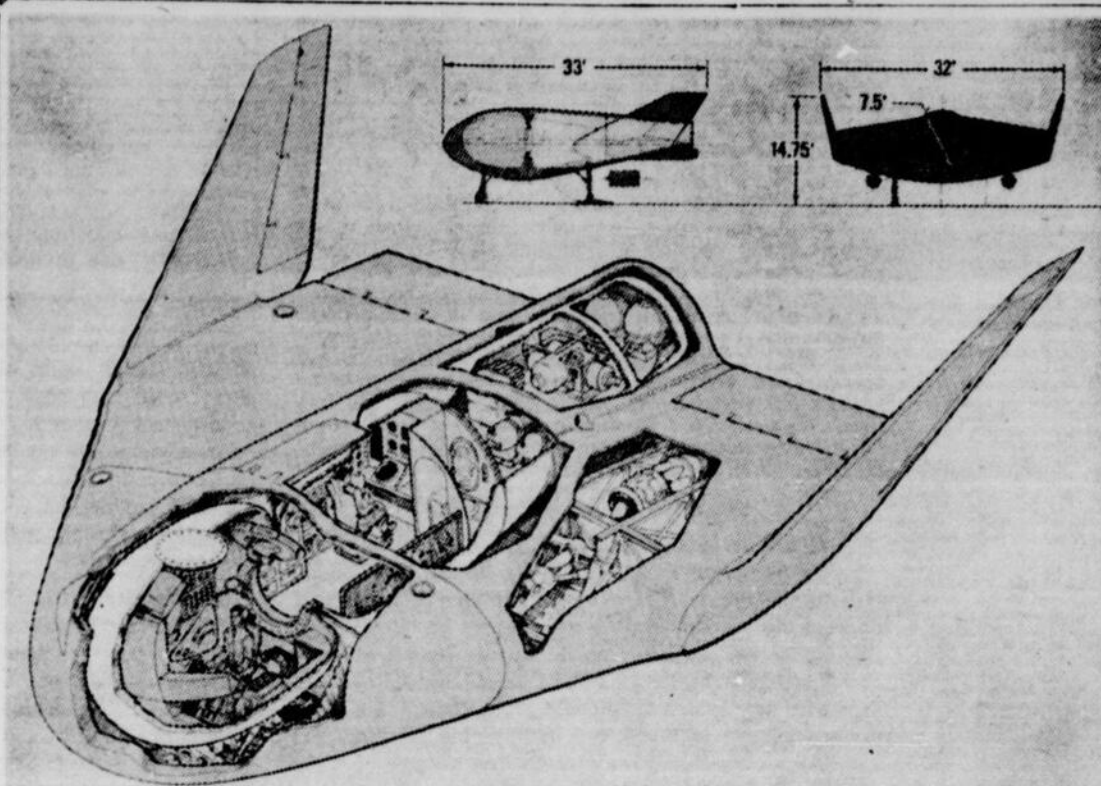
Le prototype d'appareil qui, dans sept ans, fera des voyages spatiaux d'un mois et plus. La partie avant est détachable et forme elle-même un véhicule autonome en cas d'urgence.
