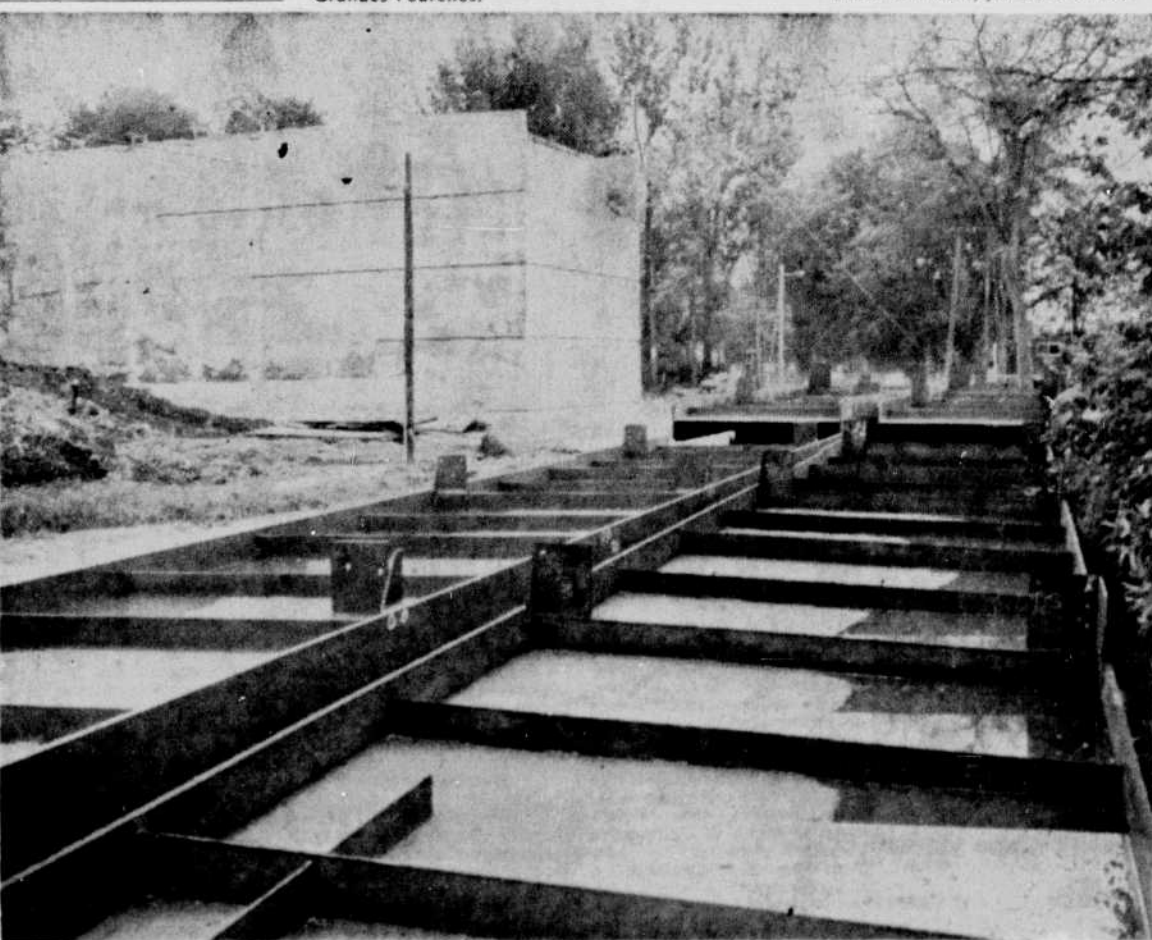
L'acier de structure du pont Montréal-Terrill, à Sherbrooke, a été transporté sur le chantier. Il s'agit de poutres de huit pieds de hauteur et de 140 pieds de longueur. Les poutres seront assemblées sur les porte-faux des
