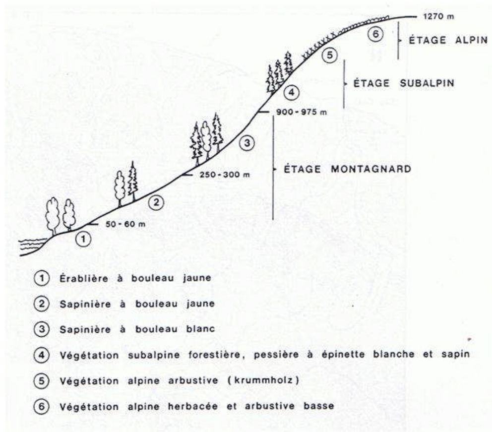
Figure 5. Étagement de la végétation entre le littoral nord-gaspésien et le sommet du mont Jacques-Cartier à 1270 m d'altitude (coupe schématique). (Source : Boudreau & Payette, 1981, dans Héту, 1998b)
