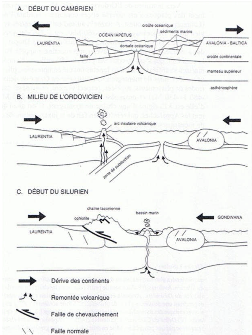
Figure 3.1 Histoire géologique des Appalaches (Hétu, 1994)
