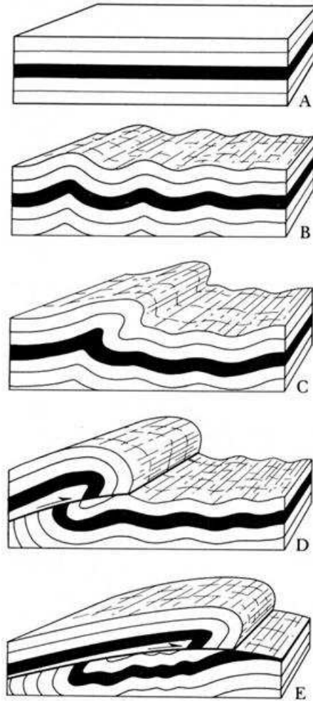
Figure 4. Évolution théorique vers le stade de nappe de charriage. A. Les couches sédimentaires non perturbées. B. Une pression latérale entraîne la formation de plis ouverts (déformations plastiques). C. La pression augmente et des plis déversés apparaissent (déformations plastiques plus prononcées). D. Apparition d'une faille inverse de chevauchement. Le seuil de résistance plastique des roches est dépassé et il y a désormais une déformation ductile. E. Nappe de charriage. (Source : USGS, 2007)
