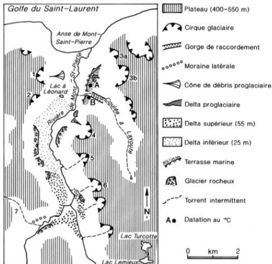
Figure 1. Croquis géomorphologique de la vallée de Mont-Saint-Pierre. (Source : Hétu et Gray, 2000)
