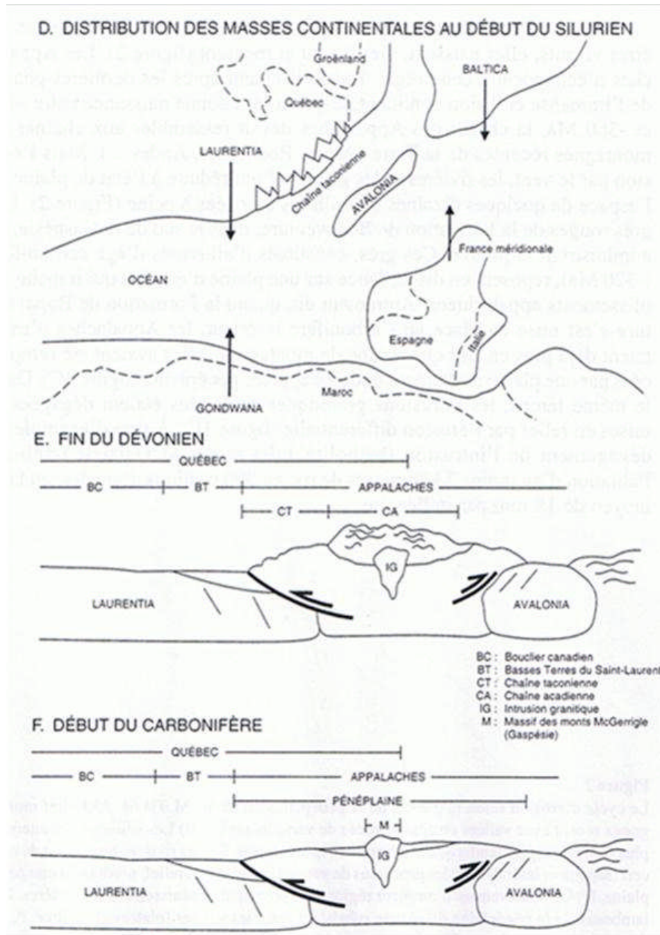
Figure 3.1 (suite) Histoire géologique des Appalaches (Hétu 1994)
