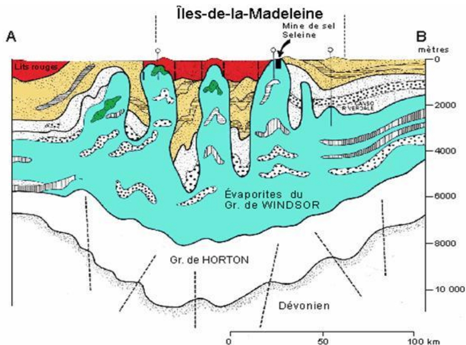
Figure 2. Coupe géologique des Îles-de-la-Madeleine. Source : Bourque (2004)
