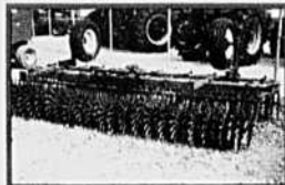
Picoteuse MW 27', repliable, avec 2 roues portées. Tag: 3657. P.S.D.
