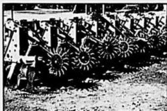
Sarclur Hiniker, 8 rangs, roue soleil. St-Guillaume. P.S.D.
