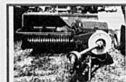
Presse à foin Vicon "461", avec lance-balles. État de neuf. Tag: 4269. P.S.D.
