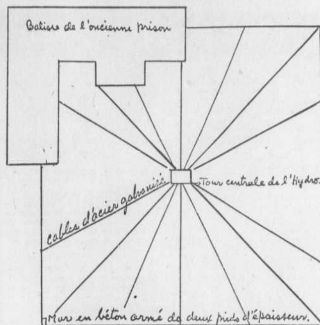
Plan du chapiteau "permanent" qui recouvrira la cour intérieure de la petite Bastille, sise sur les plaines d'Abraham; les frais encourus par la construction de ce toit se chiffrent à $150,000 et la toile coûterait à elle seule $105,000. Ce graphique est présenté en annexe d'un rapport concernant l'organisation de la "Semaine de la chanson québécoise" qui aura lieu en août prochain dans la Vieille Capitale et dont LE DEVOIR a obtenu copie.
