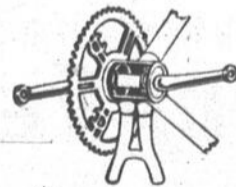
PÉDALIER C.C.M.
