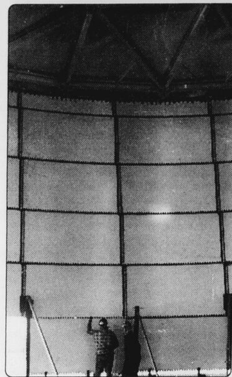
Le nouveau réservoir a 64 pieds de diamètre par 32 pieds de haut et sa capacité sera de 750 000 gallons, pouvant au besoin être portée à 1 million de gallons.
