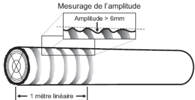
Figure 71 – Mesurage et étendue du fil ondé
