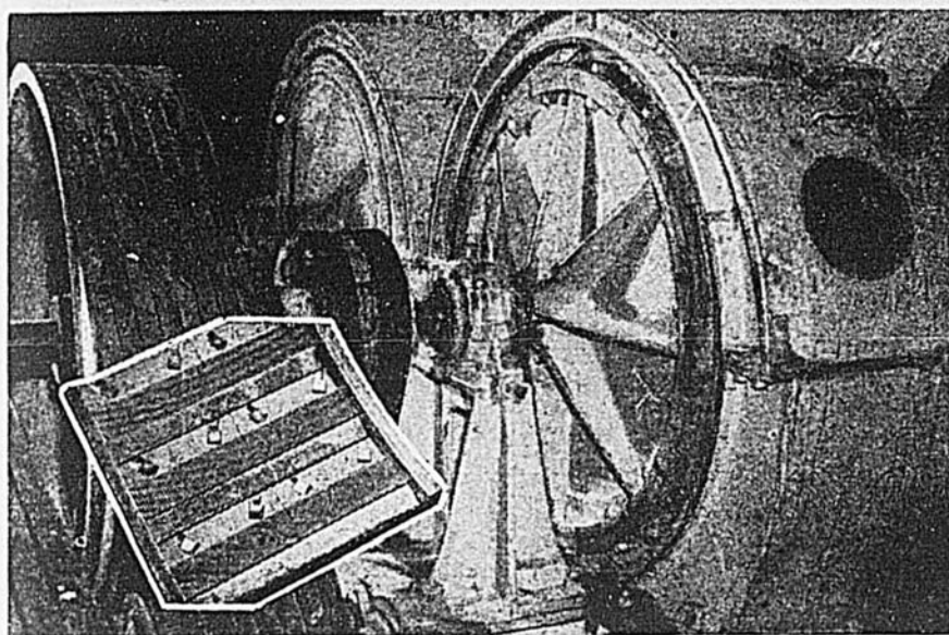
Le broyeur coupe au rythme de 50 tonnes à l'heure les betteraves en petites lanières qui ressemblent à des patates frites. Le travail se fait par la pression des betteraves sur des couteaux dont on voit un échantillon dans la petite photographie insérée.
