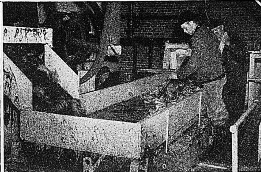
La betterave entre dans l'usine, elle est débarrassée de ses tiges, des herbes et lavée. De la cuve de lavage elle passe à la table de sélection où les dernières pierres et autres matières étrangères sont enlevées. Elle monte ensuite au broyeur.
