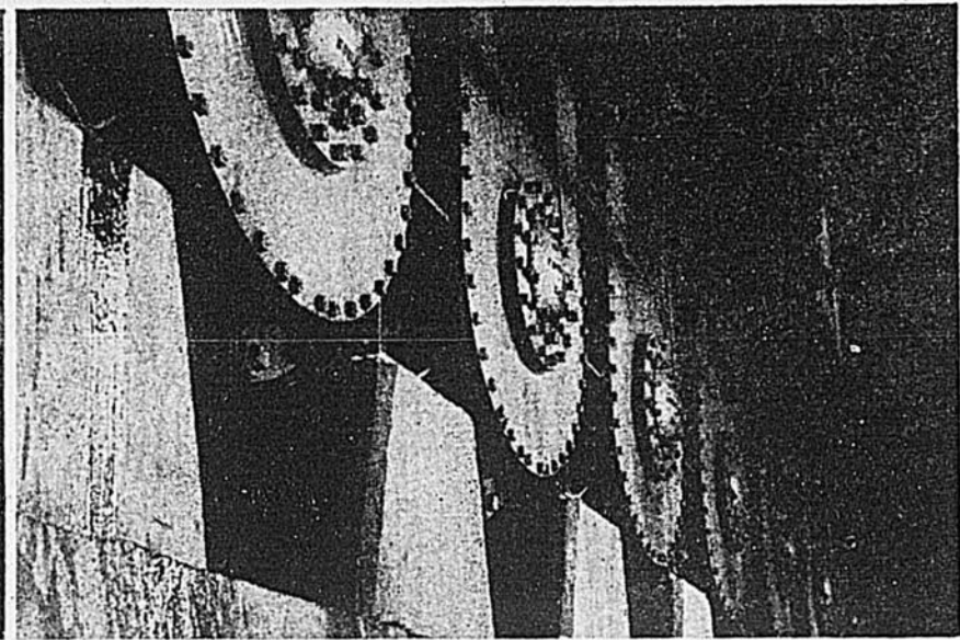
La betterave lavée, tranchée, passe dans la batterie de diffusion continue qui se compose de vingt cylindres dont quelques-uns apparaissent ci-dessus. Dans ces cylindres l'eau chaude extrait le sucre des tranches de betteraves et forme un jus épais.
