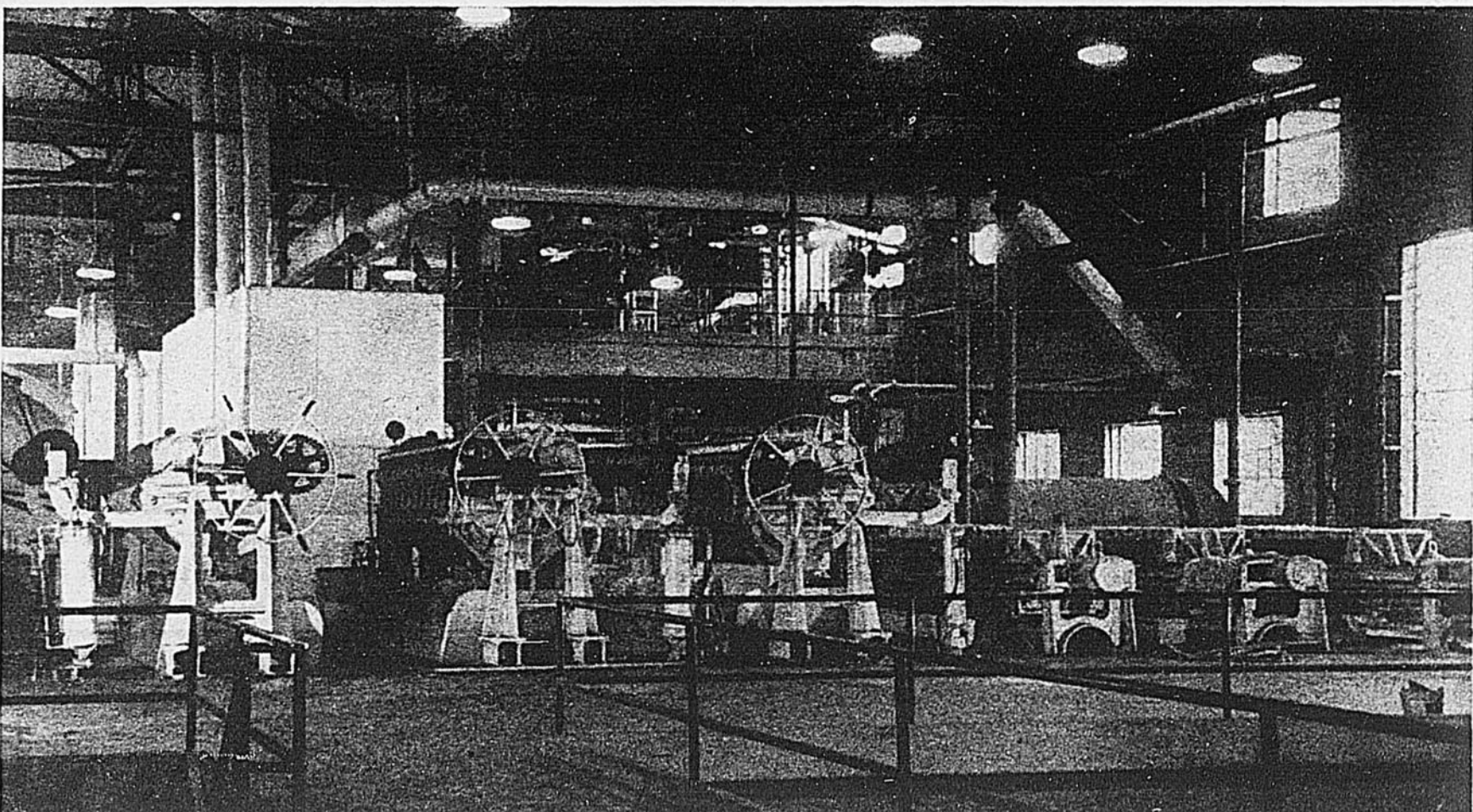
En sortant de la batterie de diffusion continue le jus passe par trois opérations différentes de clarification et de purification. Après chaque traitement le jus est soumis à une chaleur intense et à une nouvelle filtration pour éliminer toutes les impuretés qui pourraient s'y trouver. Ces opérations se font dans la machinerie que l'on voit ci-dessus.
