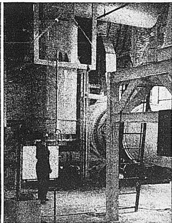
On voit ici un opérateur vérifiant la pureté du sirop épais avant qu'il ne se dirige vers la cuve d'amalgamation.
