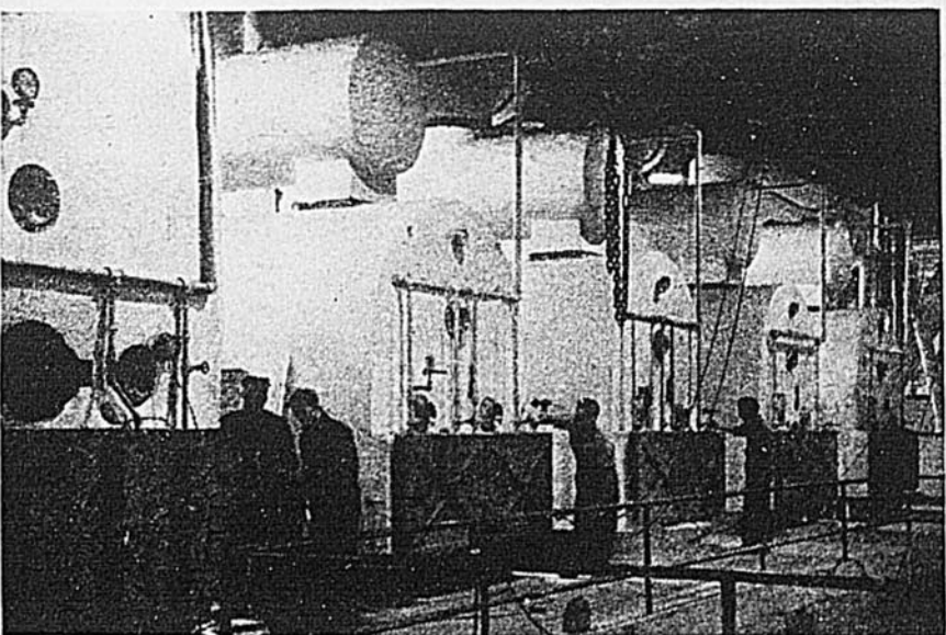
Après la clarification, le jus, devenu clair, se dirige vers les évaporateurs où l'eau en est enlevée et où le jus est concentré. Le sirop passe dans cinq évaporateurs différents où la chaleur varie de 130°F. à 230°F.
