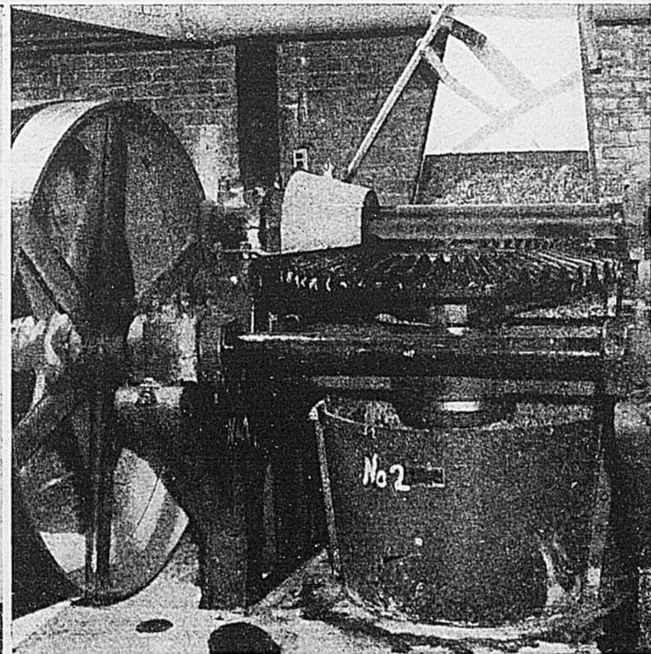
En quelques minutes, la betterave passe dans le pressoir qui en soutire toute l'eau. Il y a cinq pressoirs de ce genre qui sont alimentés par un conduit général.
