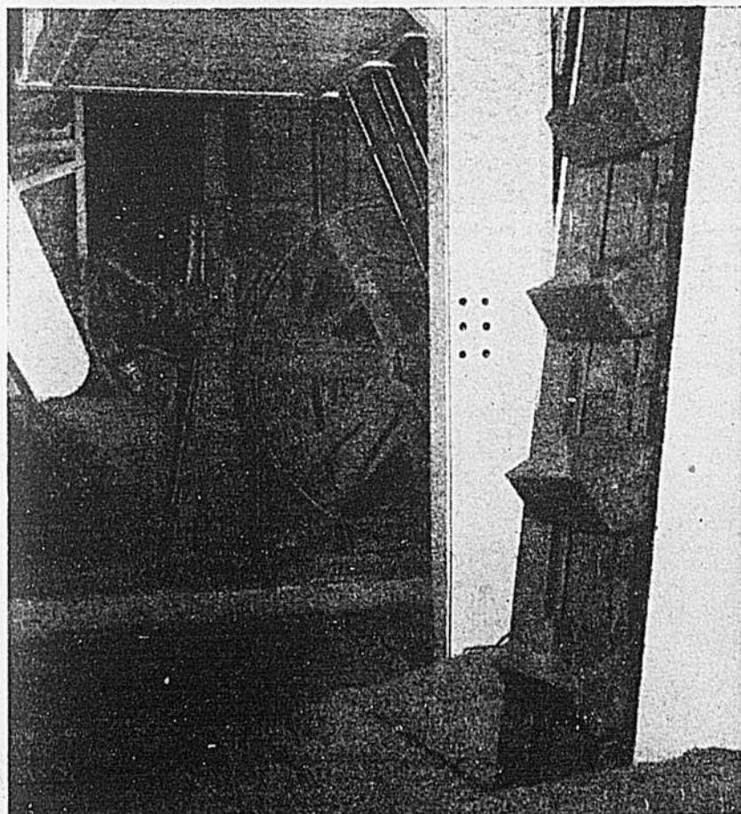
Le déchet de la betterave est ensuite envoyé de la batterie de diffusion au pressoir par un ascenseur à godets. Là encore, le travail est automatique.
