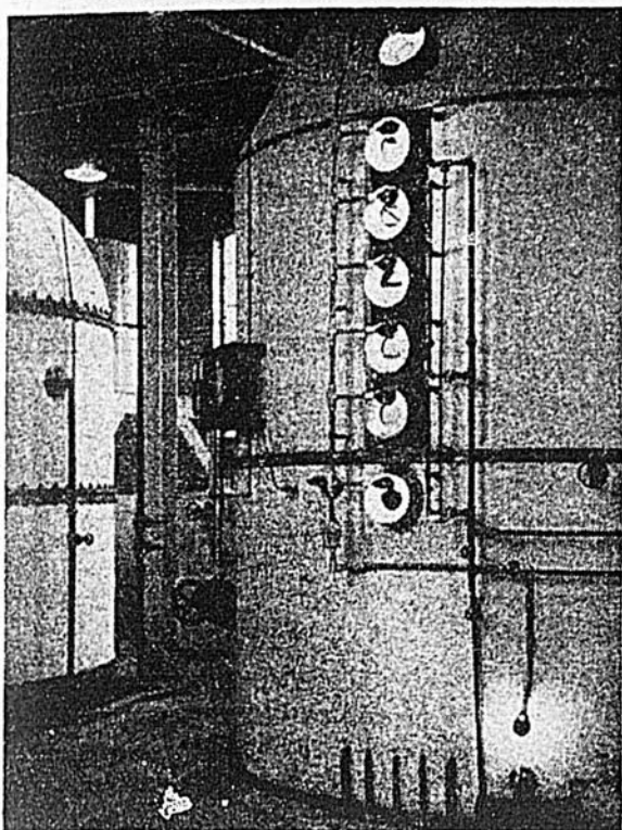
Voici la cuve d'amalgamation où le sucre est cristallisé sous la forme qu'on achète le sucre granulé. Le sirop est bouilli à une chaleur de 165°F. à 175°F.
