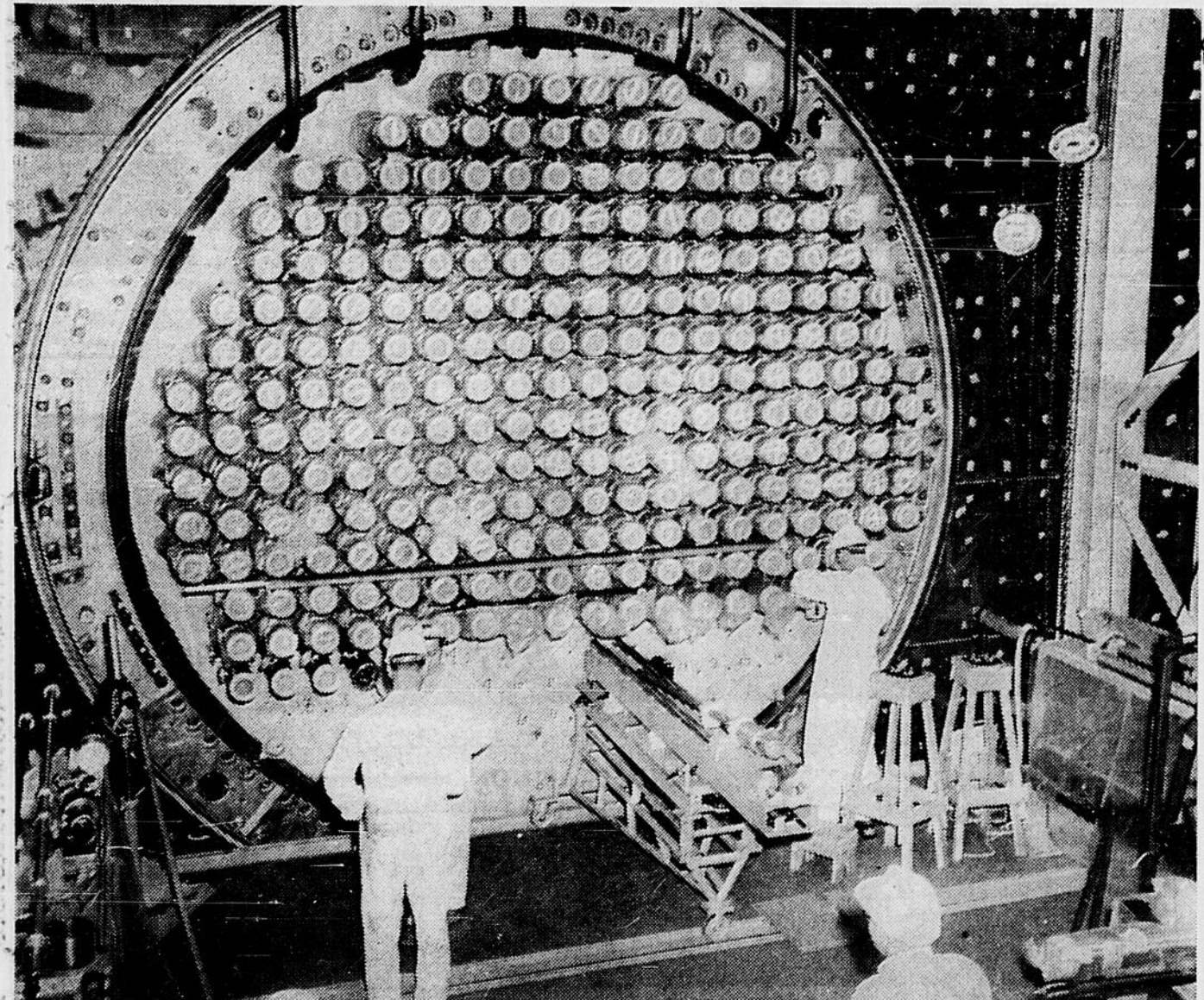
PARACHEVEMENT PREVU EN 1965 — Des techniciens installent des tubes de refroidissement à l'extrémité du réacteur de la centrale d'énergie nucléaire de Douglas Point, localité située à 130 milles au nord-ouest de Toronto. Cette
