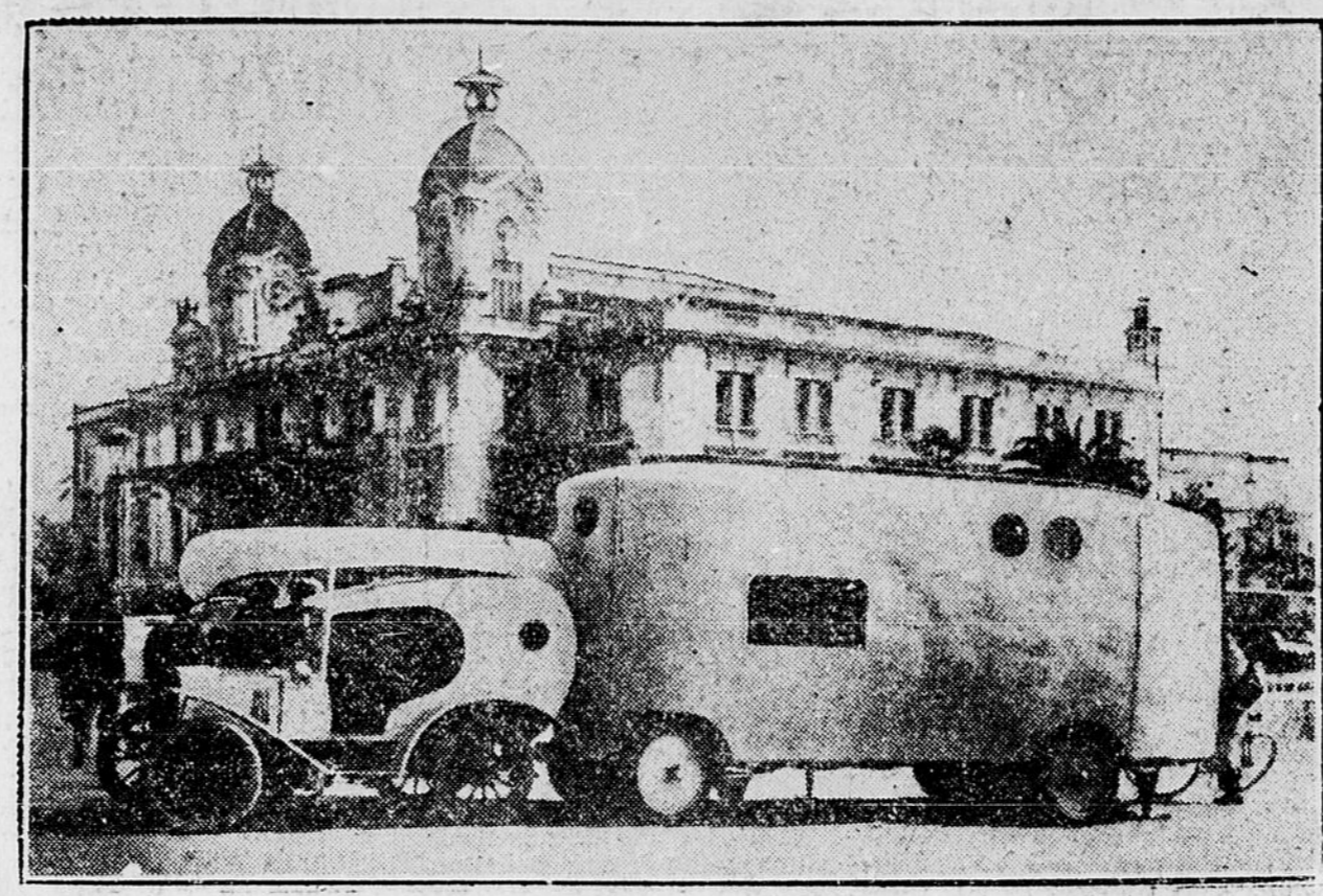
UN RECENT SPECIMEN DES VEHICULES AVEC LESQUELS IL EST POSSIBLE DE TRAVERSER LES DESERTS. La force motrice de cet appareil vient du petit auto que nous voyons à l'avant. La grande maison roulante sert de gîte aux touristes. Toutes les choses nécessaires à une semblable traversée sont renfermées dans cette maison roulante. On voit sur le toit du petit auto un canot.
