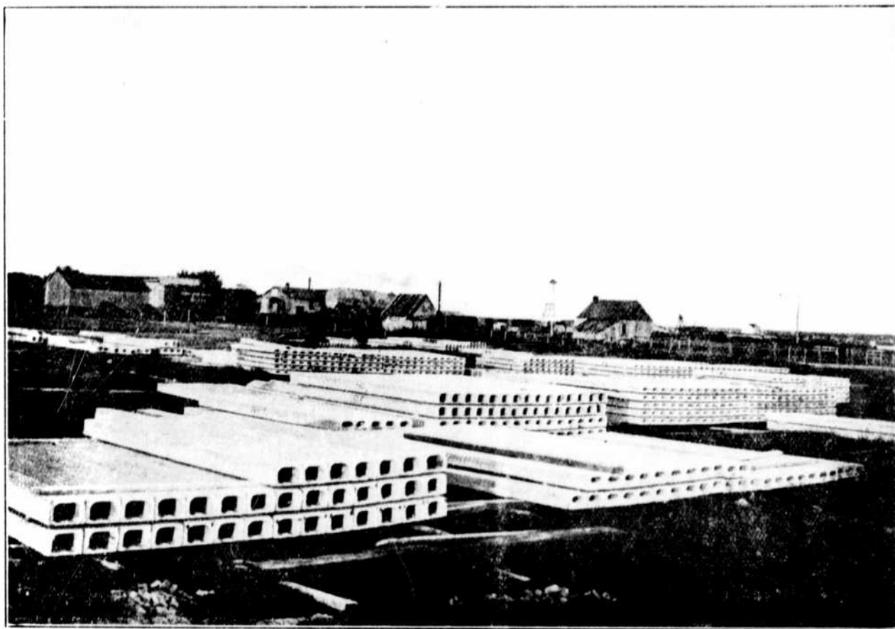
ETABLISSEMENT DE THE CANADIAN SEIGWART BEAM CO., LTD.
