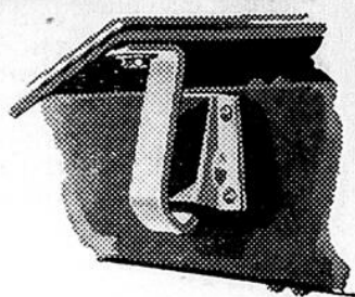
Les nouveaux éléments de montage amortissent efficacement les vibrations. D'où plus de confort et durée prolongée de la cabine. (Séries 920-980.)
