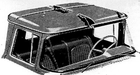
La construction à double paroi donne une grande rigidité aux panneaux du toit et de la partie supérieure de la cabine: protection et isolation supérieures.
