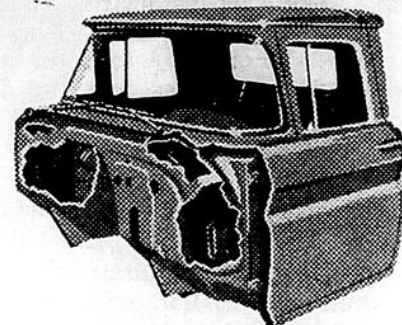
L'avent à double paroi procure une résistance exceptionnelle. Il sert également de chambre d'air pour le système de chauffage.
