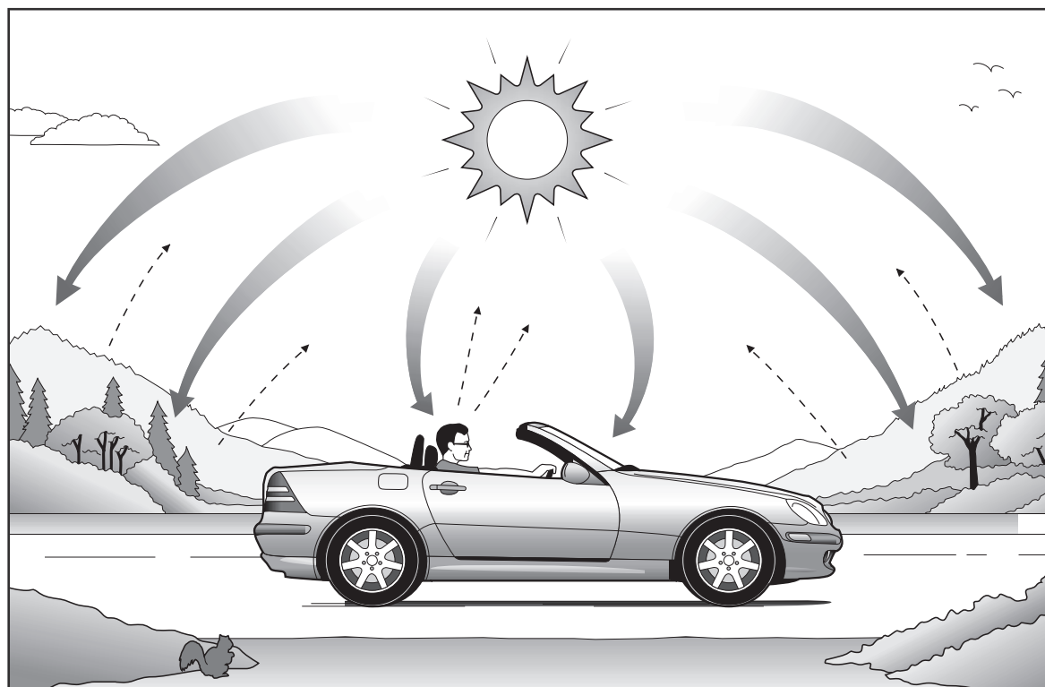
Schéma 1. Photosynthèse et respiration.
