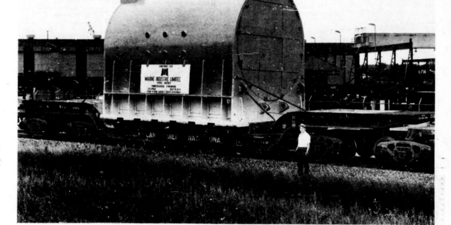
COMPENSATEURS DE GRANDE PUISSANCE POUR L'HYDRO-QUEBEC - Le premier des quatre compensateurs synchrones pesant 350 tonnes et construit pour le compte de l'Hydro-Québec quitte les ateliers de Marine Industrie Limitée, Soré, en destination du poste Duvernay, près de Montréal.
