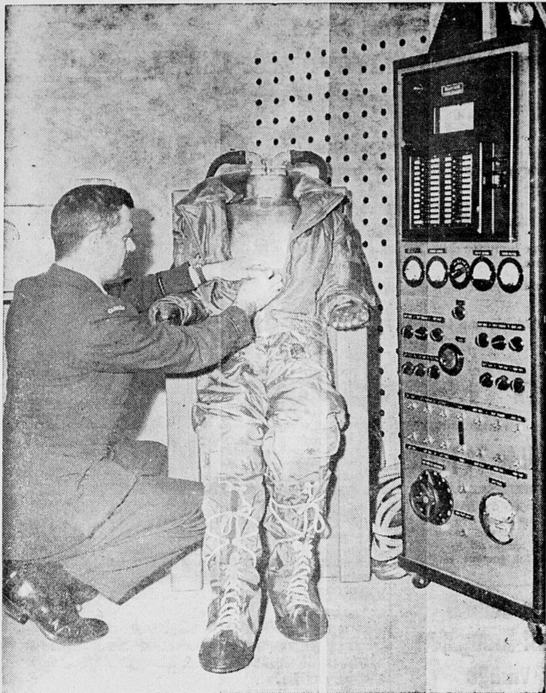
Avant de procéder à une série d'expériences, on revêt l'homme de cuivre et un vêtement de protection. Ce mannequin permet aux chercheurs d'Institut de médecine aéronautique de poursuivre des expériences relatives à l'ambiance atmosphérique et aux vêtements de protection.
