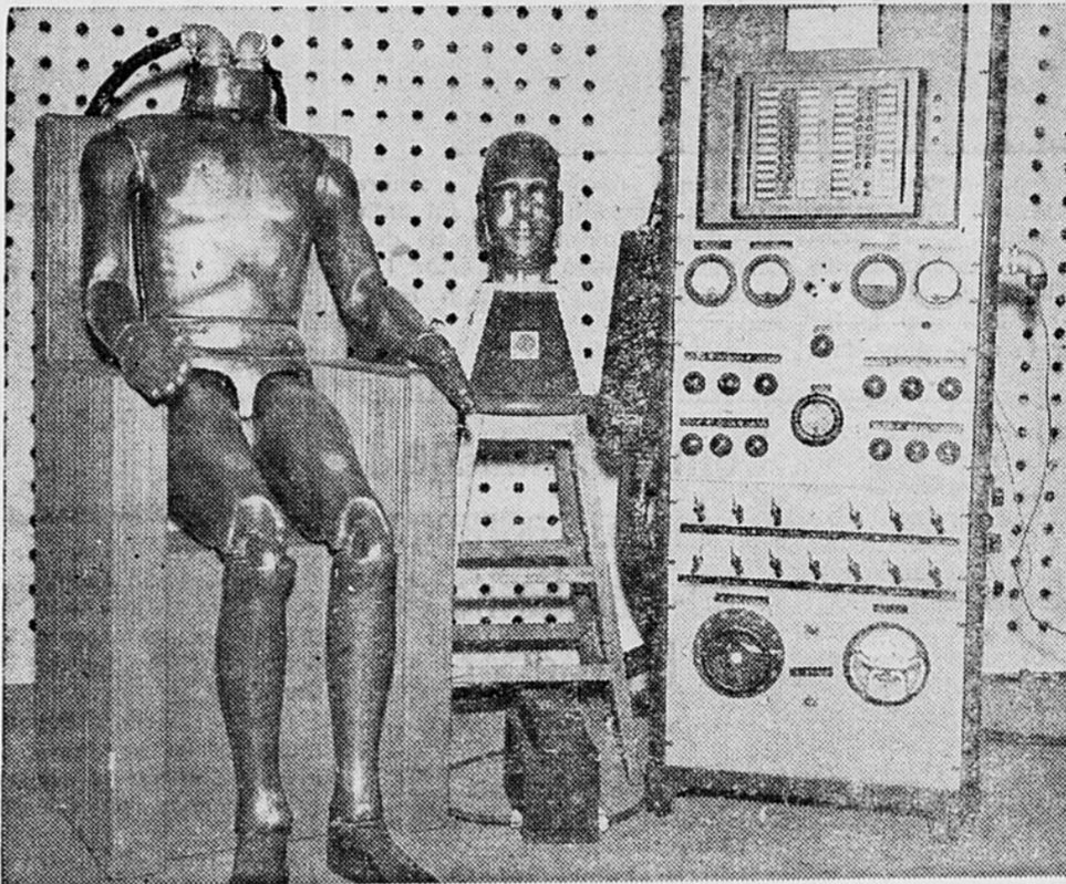
L'homme de cuivre est articulé, ce qui lui permet d'adopter différentes poses lors des expériences. Sur cette photo, on peut voir la machine de contrôle, à droite du siège qui sert de support au mannequin. Celui-ci peut être soumis à des températures et à des efforts extrêmes qui pourraient être dangereux pour l'organisme humain.
