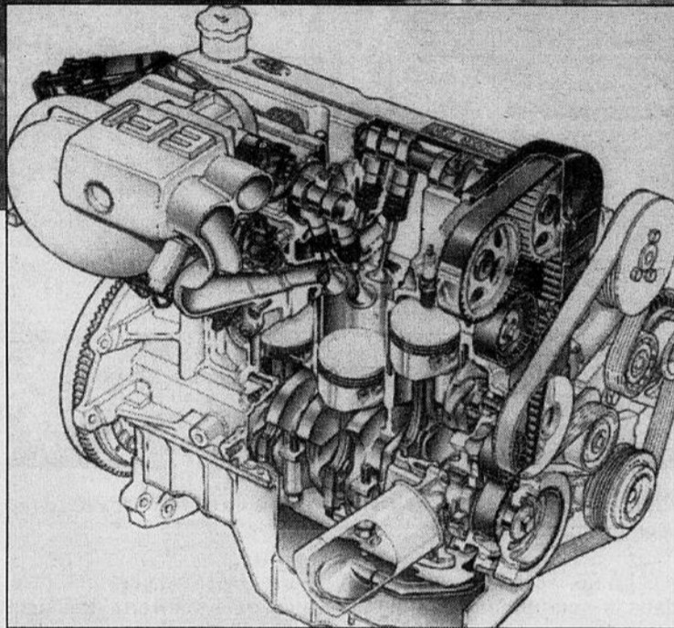
Des composantes, dont le moteur quatre cylindres, vu à gauche, de la Ford Escort XR3i anglaise, disponible en Europe, pourraient bien se retrouver prochainement dans les produits Ford américains. Pour les essais, notre chroniqueur a bénéficié d'une voiture équipée du 1,8 litre développant 105 chevaux-vapeur.
