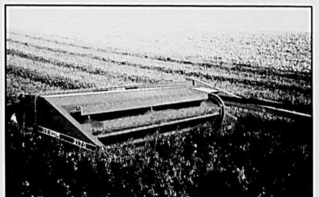
Faucheuse-conditionneuse conventionnelle.
