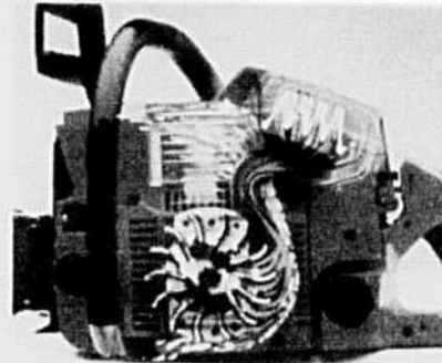
Système à injection d'air Husqvarna
