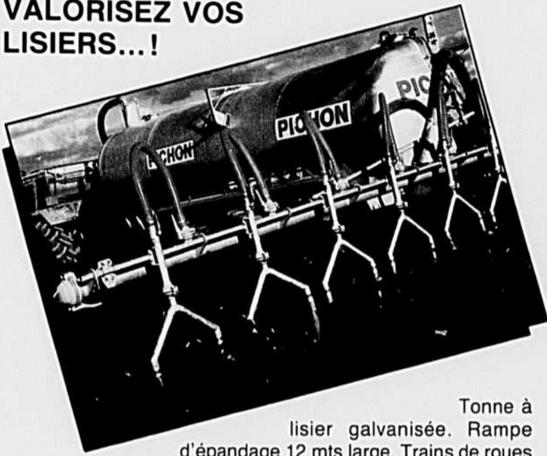
Enfouisseur: évite les pertes d'azote.
