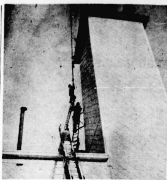
Une autre antenne. — A la suite des dommages causés par la foudre, on devra changer la longue antenne du système de radiopole d'Asbestos. C'est pourquoi les employés municipaux ont descendu l'antenne hors d'usage qui sera remplacée par une plus courte qui sera installée sur la tour de l'hôtel de ville. Ainsi en ont décidé les édiles municipaux lors d'une réunion spéciale en comité. (Photo La Tribune, par Marcel Charette, Asbestos)
