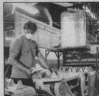
Le chauffage à hyperfréquences et les transporteurs automatisés utilisent l'énergie de façon plus productive pour MBM Ceramics.
