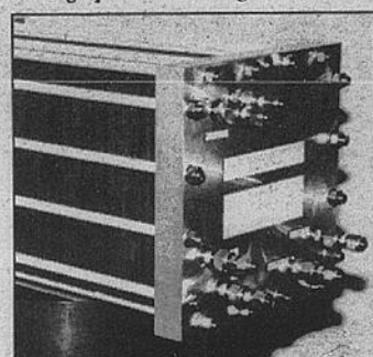
Une cellule électrochimique à polymère solide transforme l'hydrogène en énergie utile pour Dow Chemical Canada.
