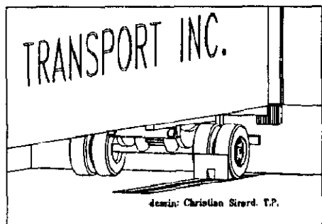
Figure 1 - Les systèmes à cale de roue
