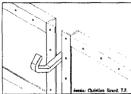
Figure 2 - Les systèmes à crochet
