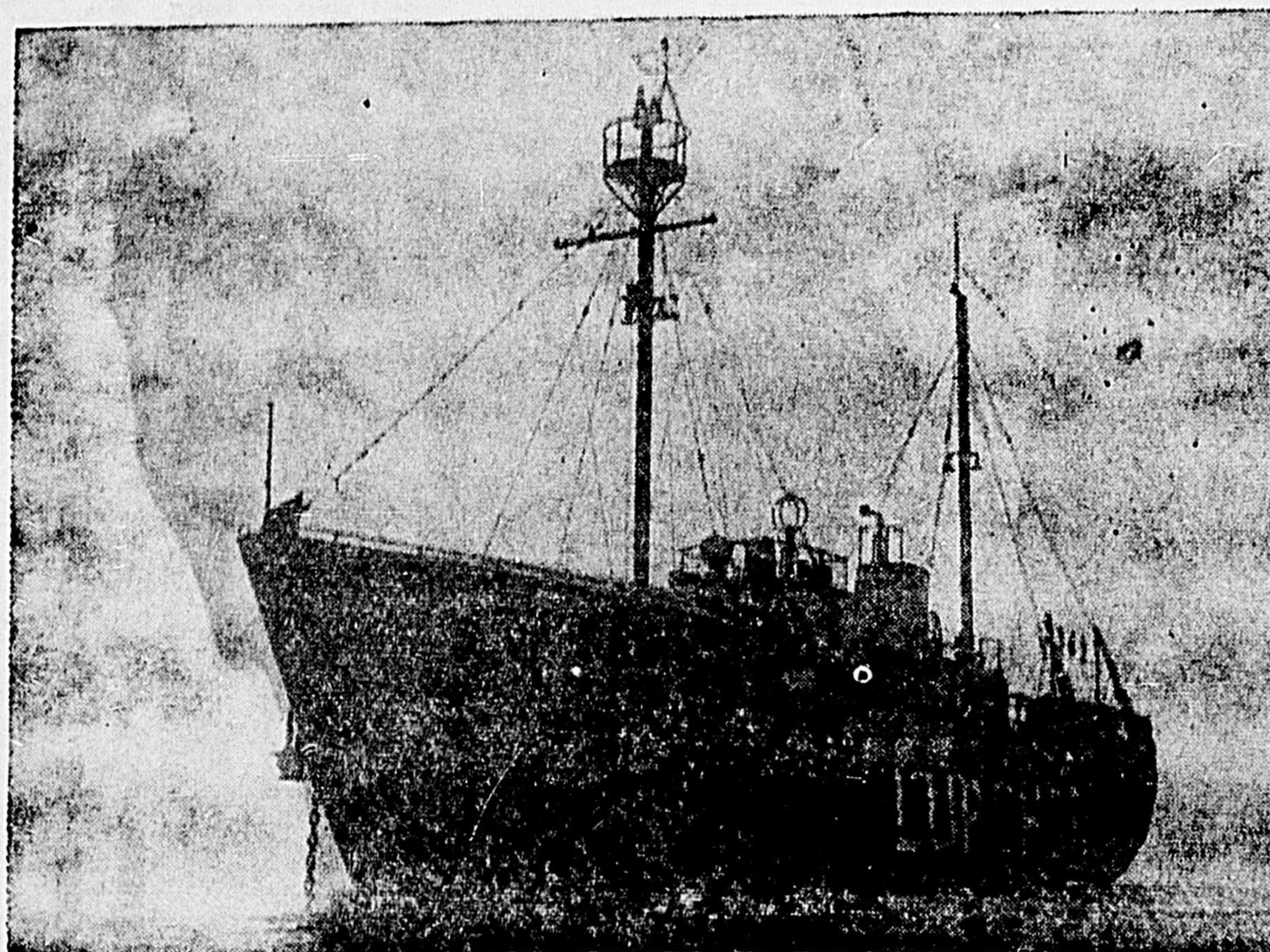
Voyez le phare au haut d'un des mats du Lurcher II qui est ancré à plusieurs milliers de pieds au large des hauts-fonds.
