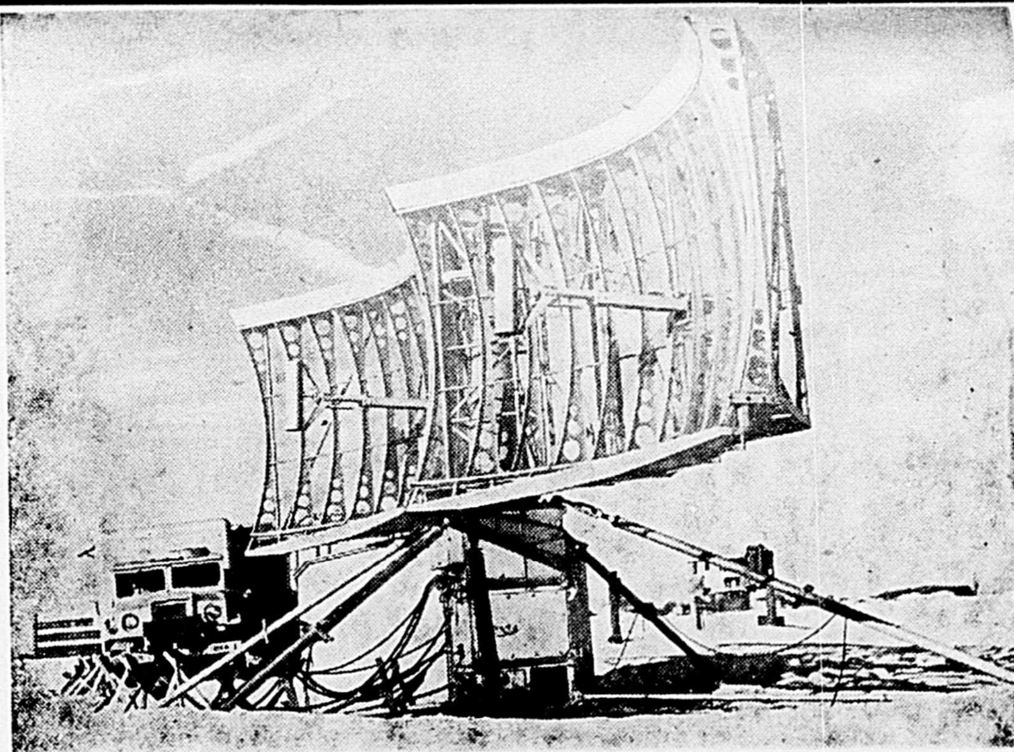
Appareil de radar
