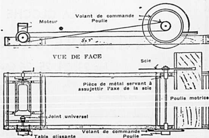
Cette scie ronde transportable est facile à construire. Remarquez que le moteur d'auto illustré ici peut être remplacé par un moteur électrique.
