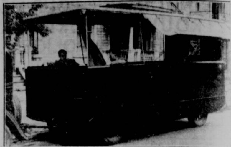
Posé sur quatre tiges de fer mues par un seul levier, le toit de la remorque peut être monté jusqu'à une hauteur de six pieds et trois pouces, à l'intérieur, ce qui la rend très pratique, comme on le voit ci-haut. (Photo "Le Petit Journal").
