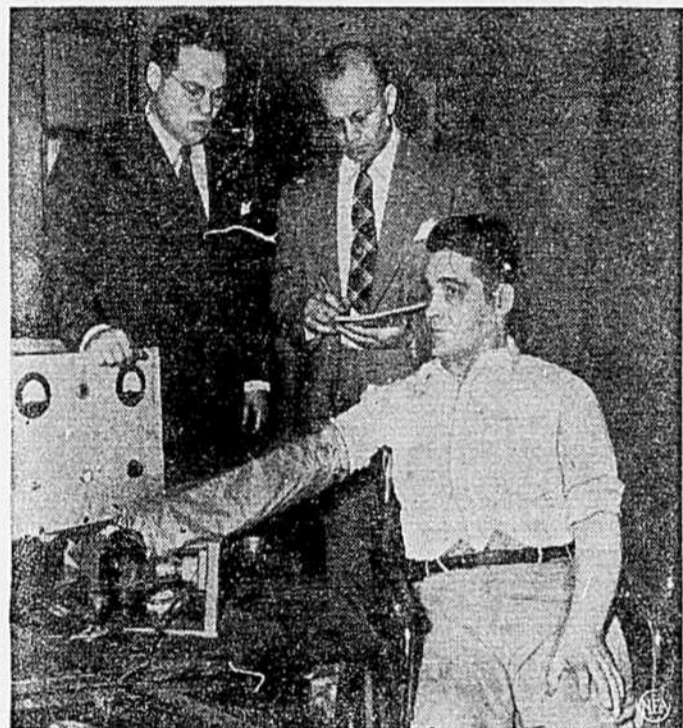
James-C. Flickinger, une victime de la paralysie infantile, travaille pour l'inventeur James-H. Rand. Il fait l'expérience d'une manche mécanique inventée pour mesurer les capacités caloriques du nouveau tissu X. Rand, à gauche, et son ingénieur, Wallace-H. Nichols, prennent des notes sur l'expérience.
