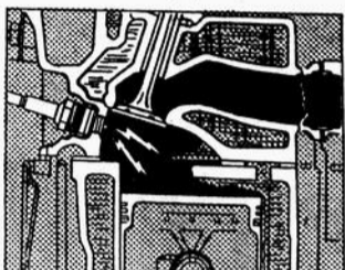
Combustion flamme bleue
